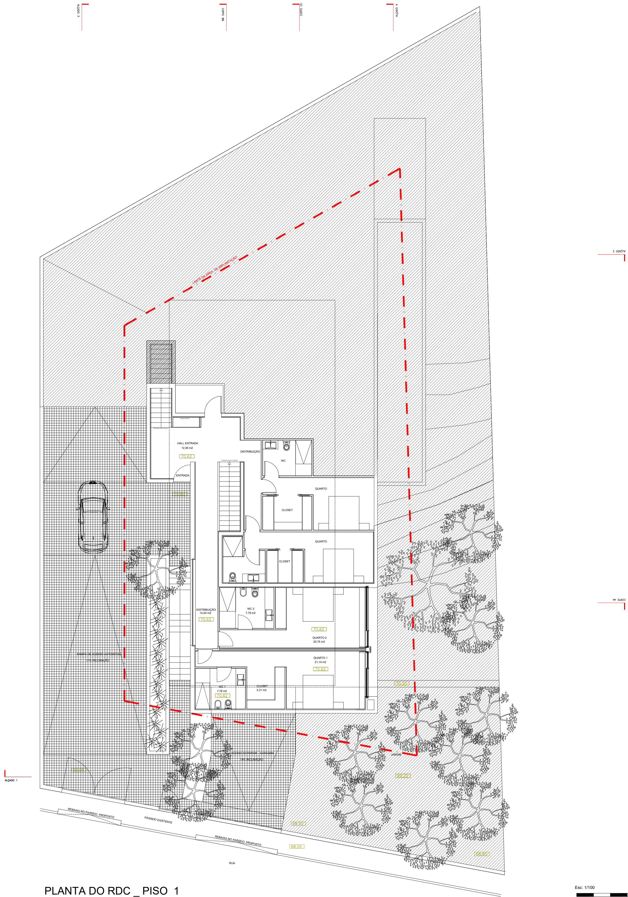
PLANTA DO RDC _ PISO 1
