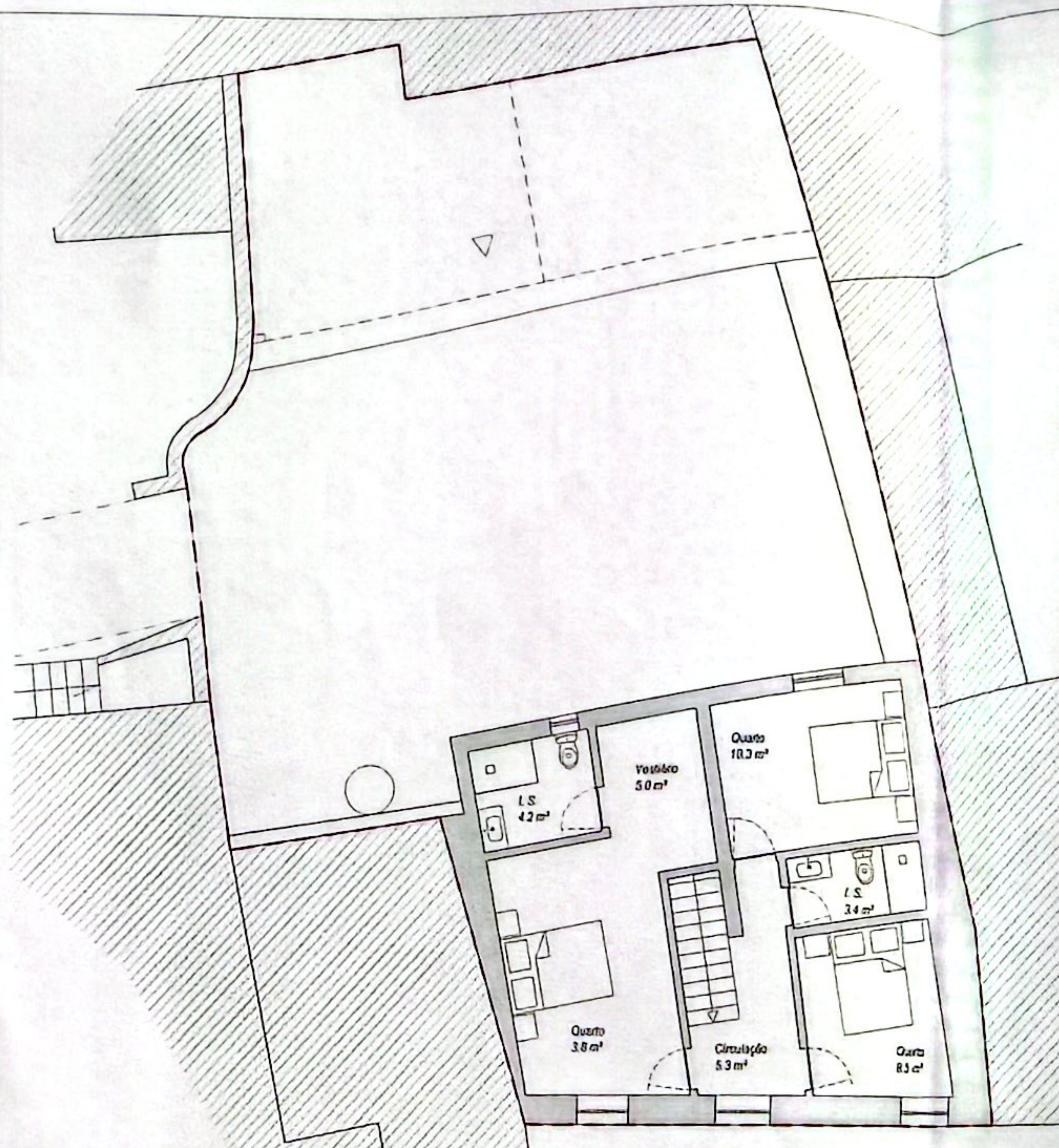
PLANTA DO PISO 2 (Andar) - apresentação
