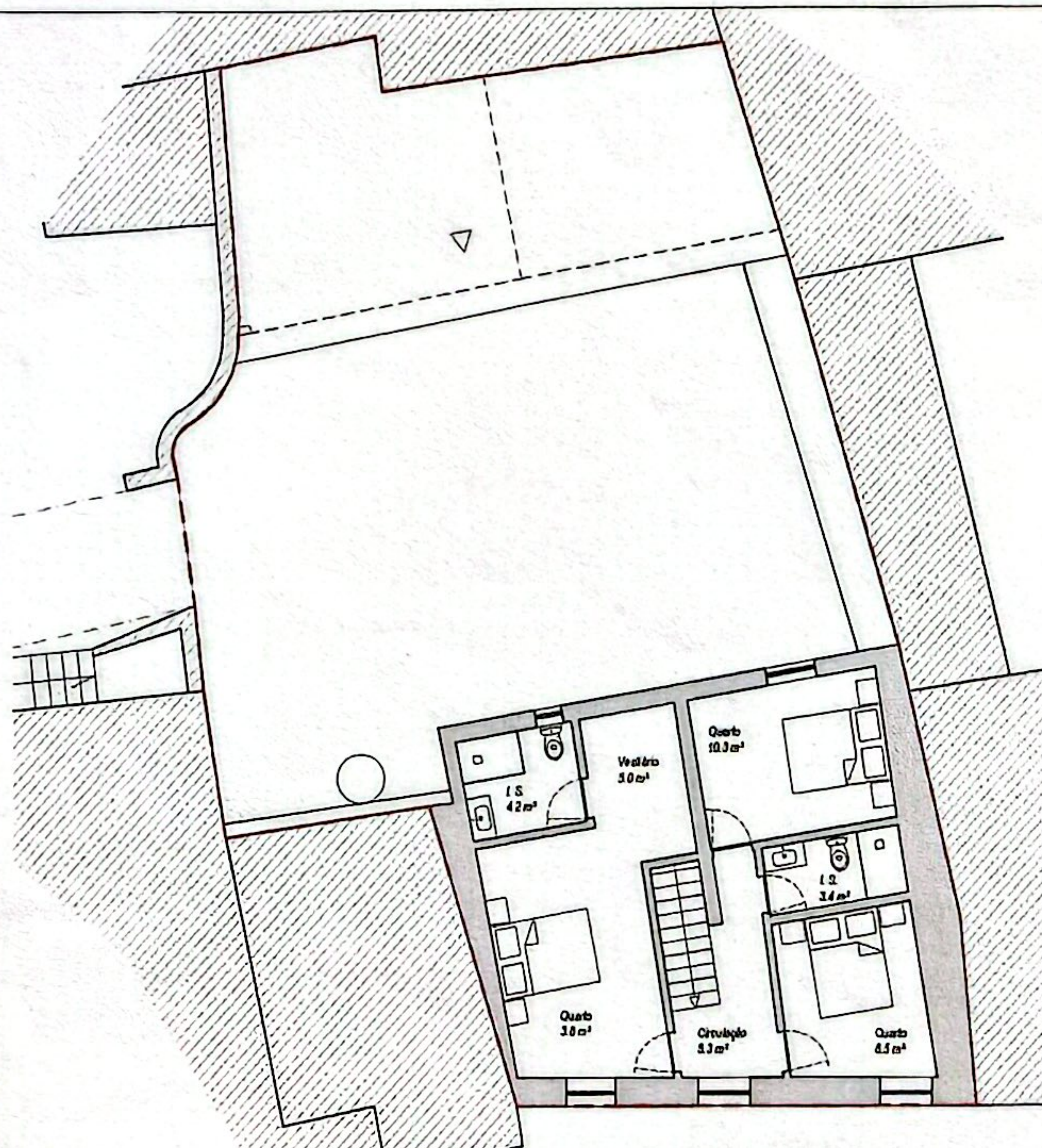
PLANTA DO PISO 2 (Andar) - apresentação
