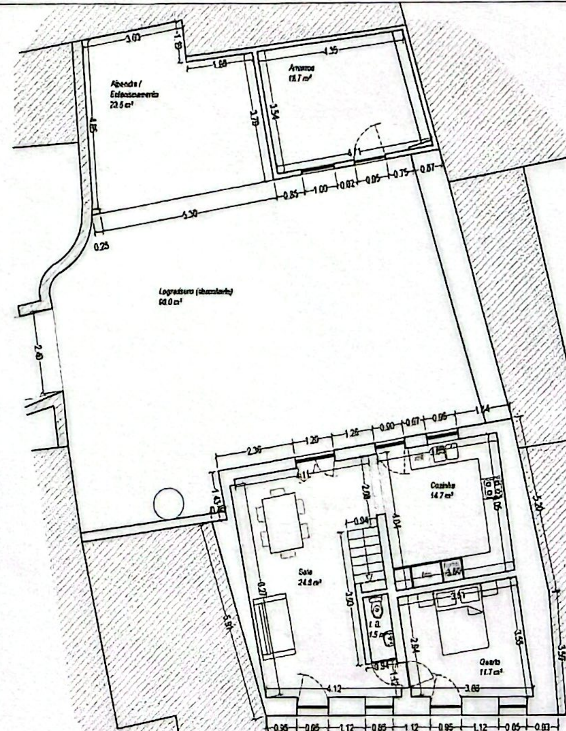
PLANTA DO PISO 1 (1º/Chão) - cotada
