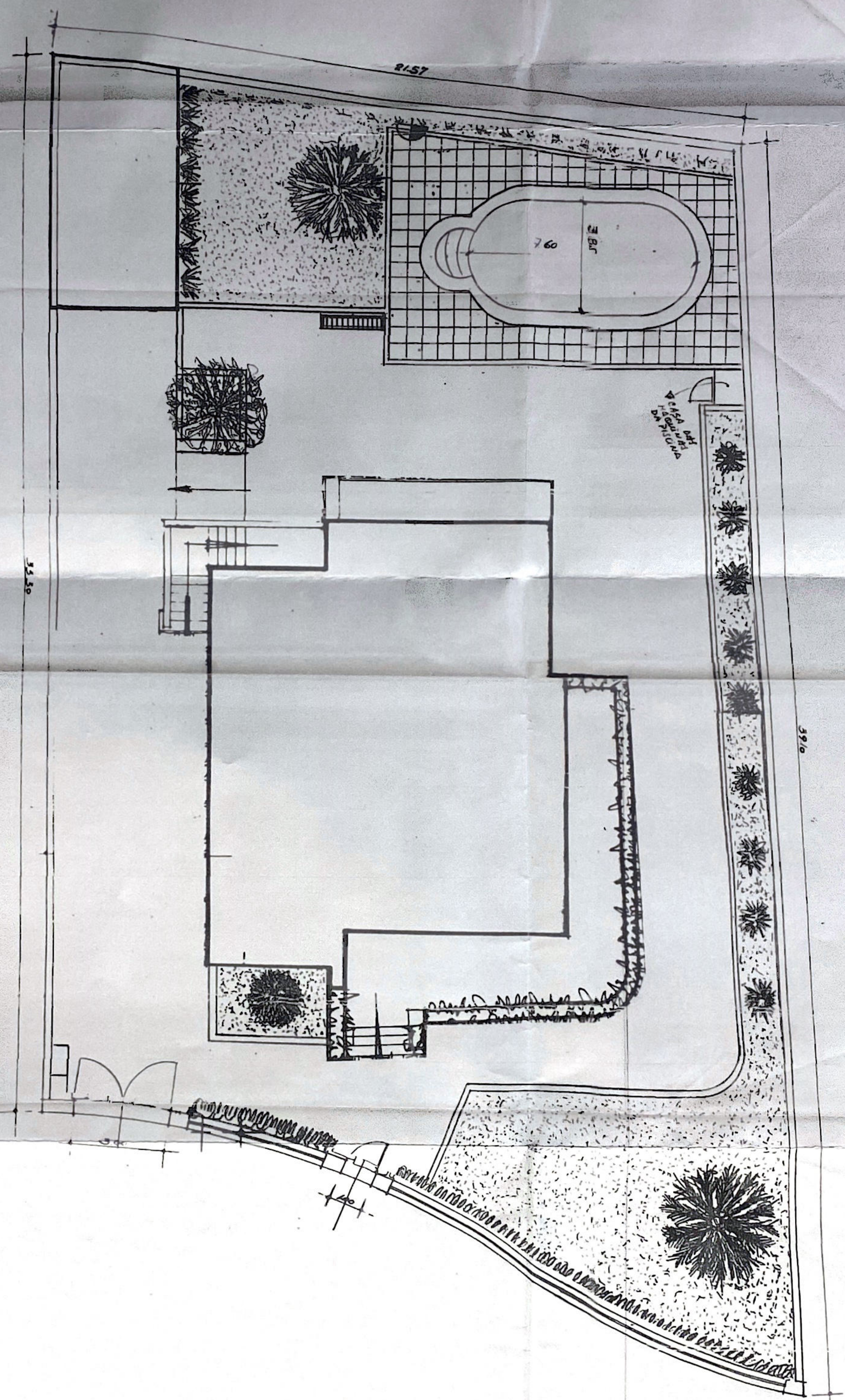
PLANTA DE IMPLANTAÇÃO
