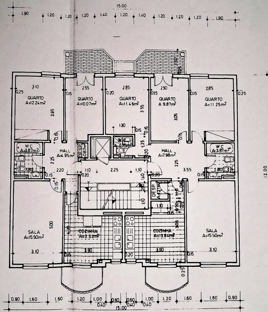
PLANTA DOS ANDARES
