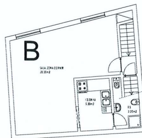
PISO 1
