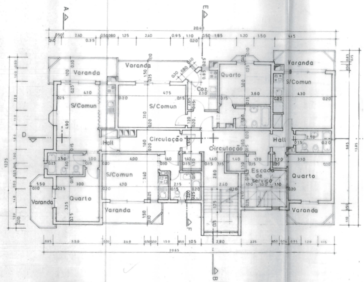
PLANTA do 2º ao 9º PISO
