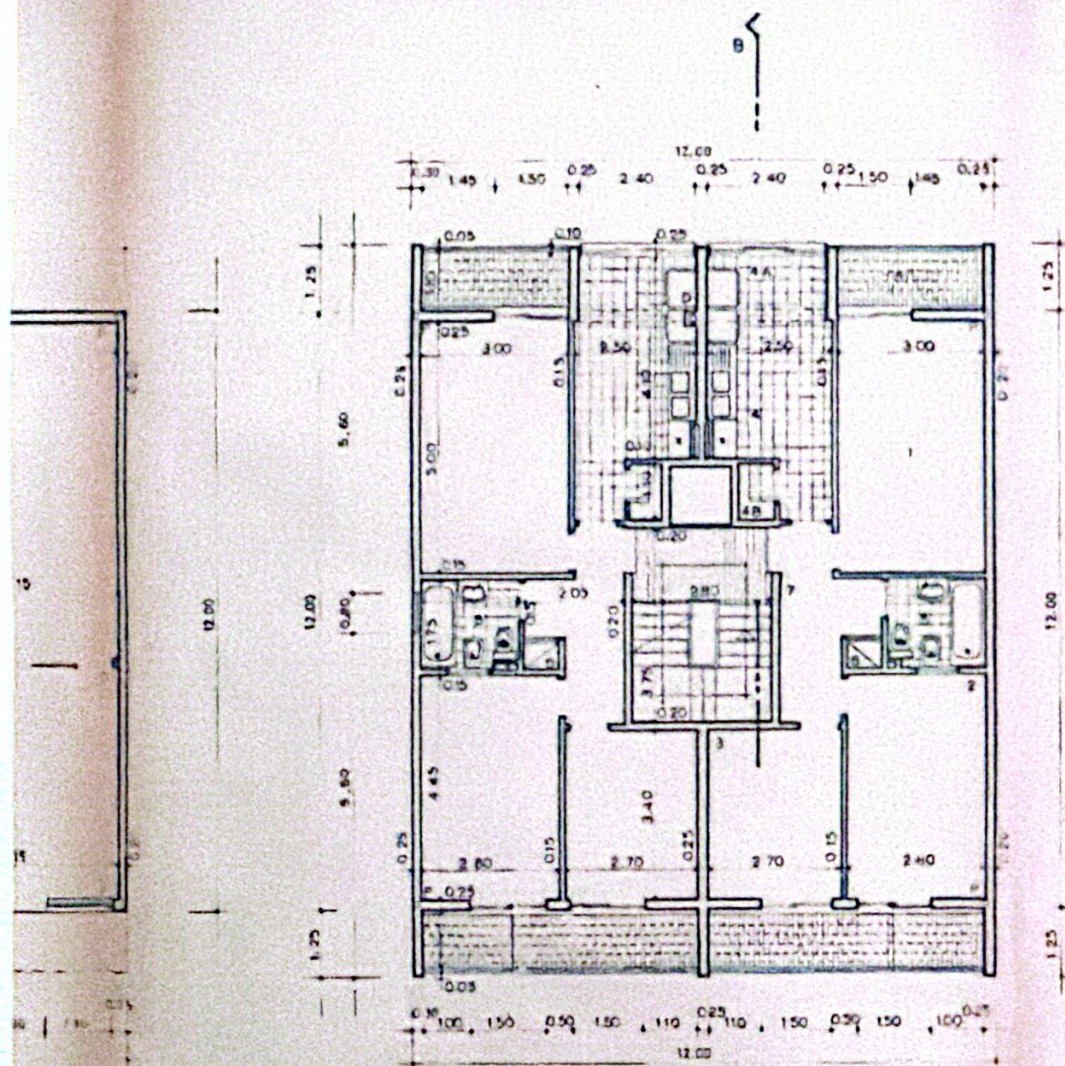
PLANTA DOS ANDARES
