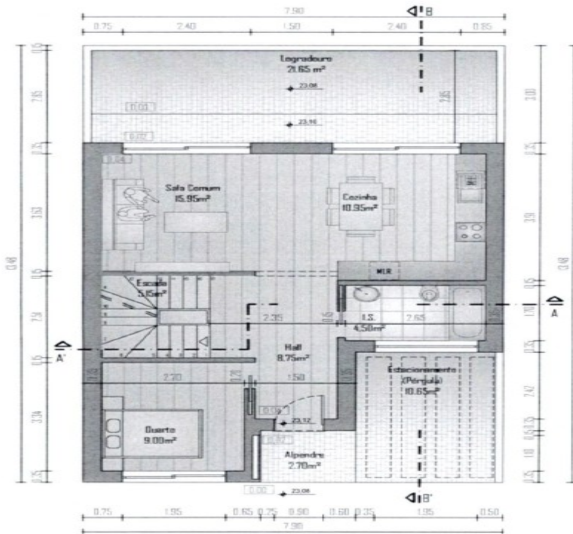
Planta do Piso I
