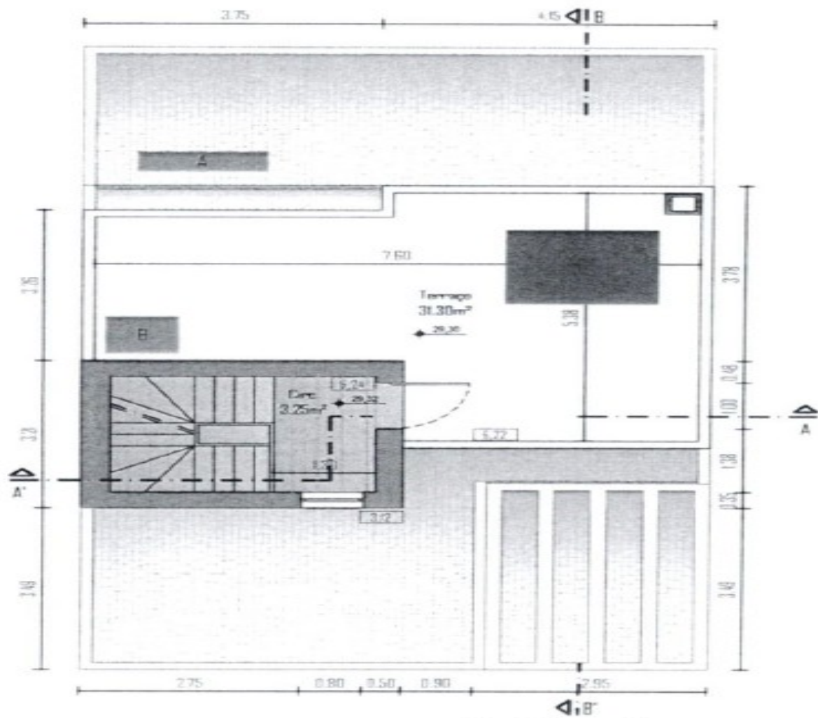
Planta de Acesso a Cobertura
