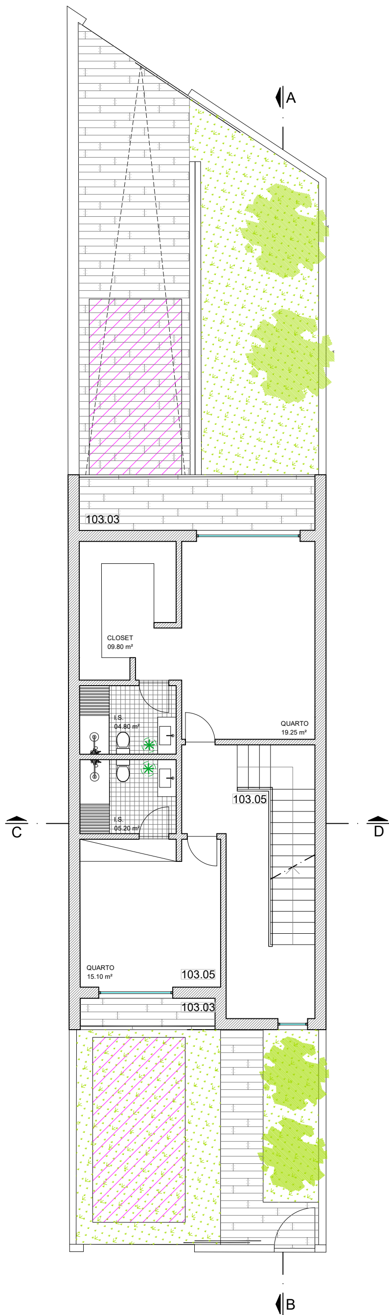
PLANTA DO 1º ANDAR
