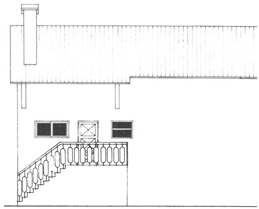
POSTERIOR
