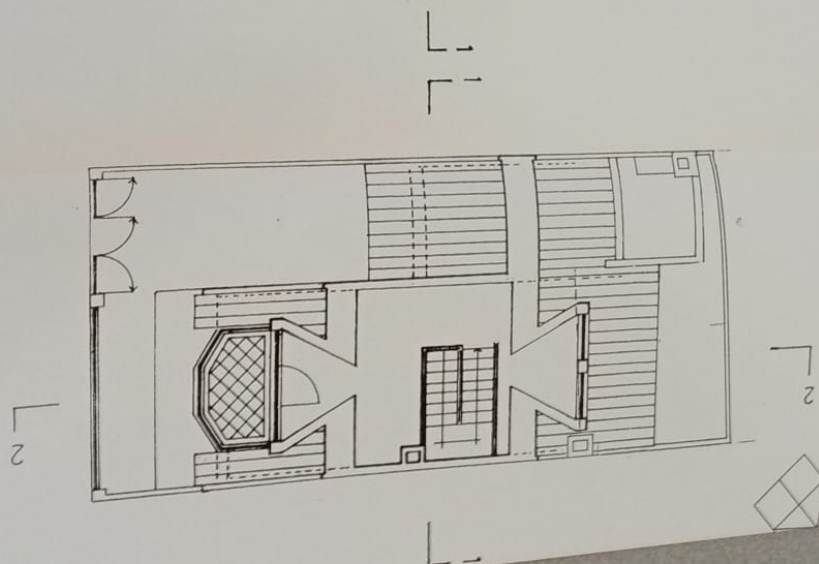
PLANTA DO PISO ÁTICO
