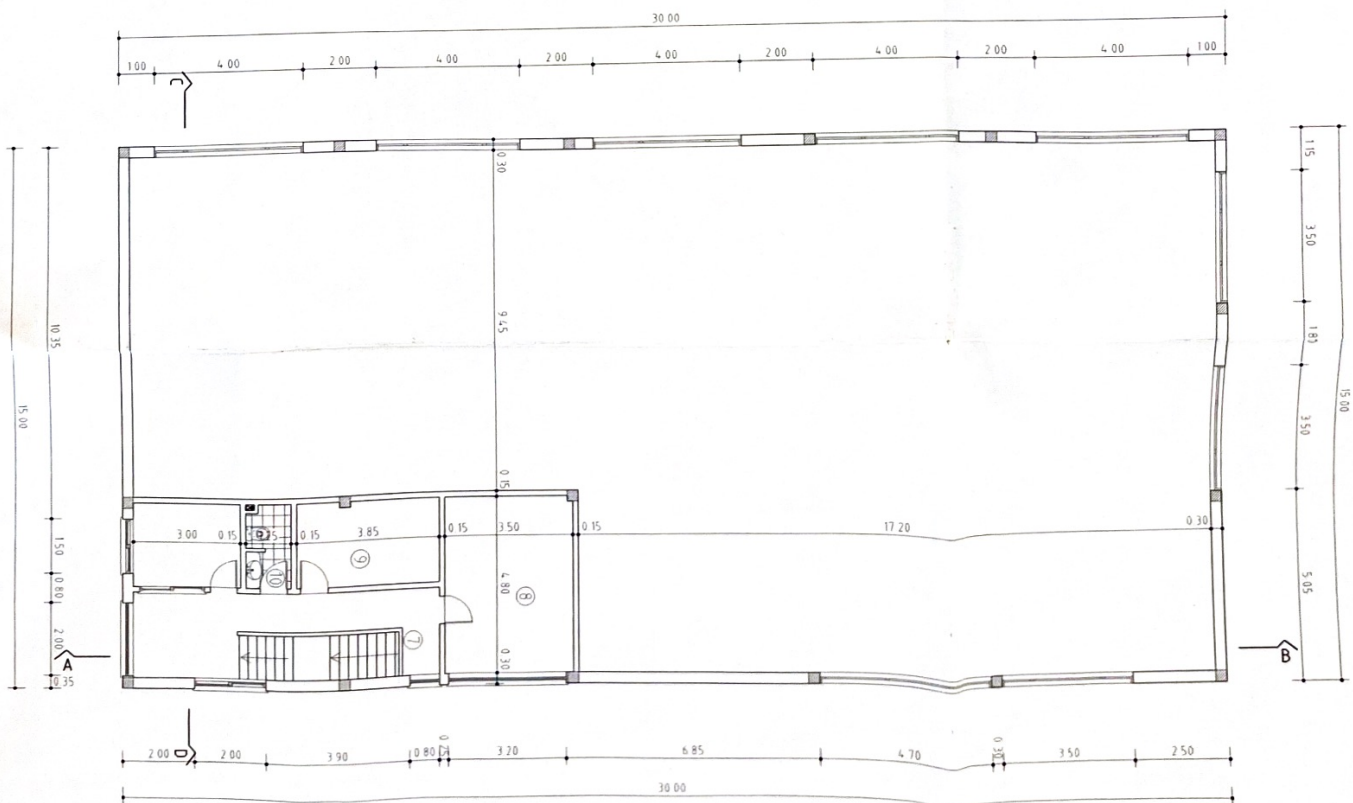
PLANTA DO 1º ANDAR
