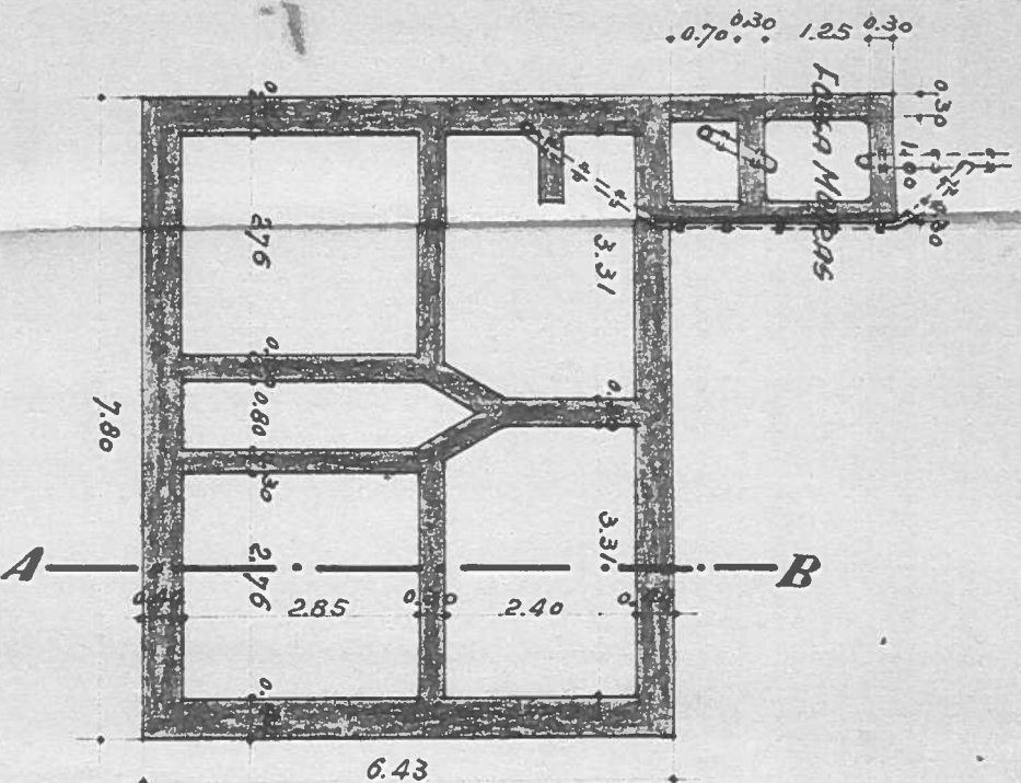
PLANTA DAS FUNDAÇÕES
