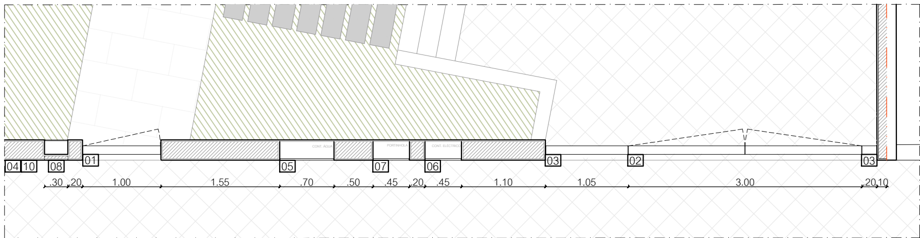
Planta - muro de entrada (escada 1:50)
