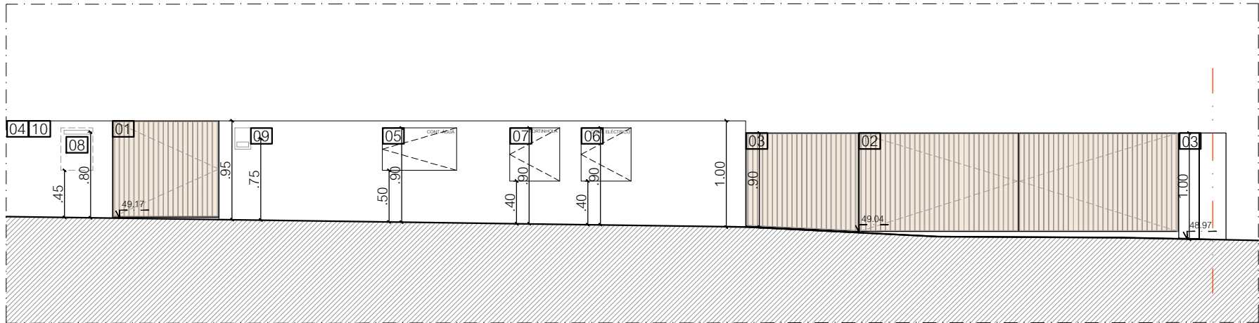
Alçado - muro de entrada (escada 1:50)
