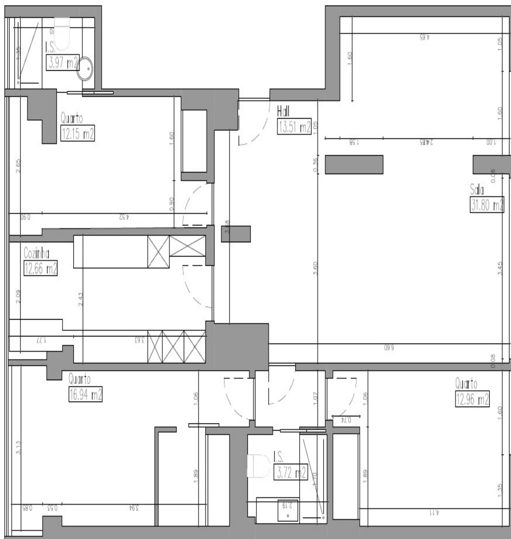
Planta T3
