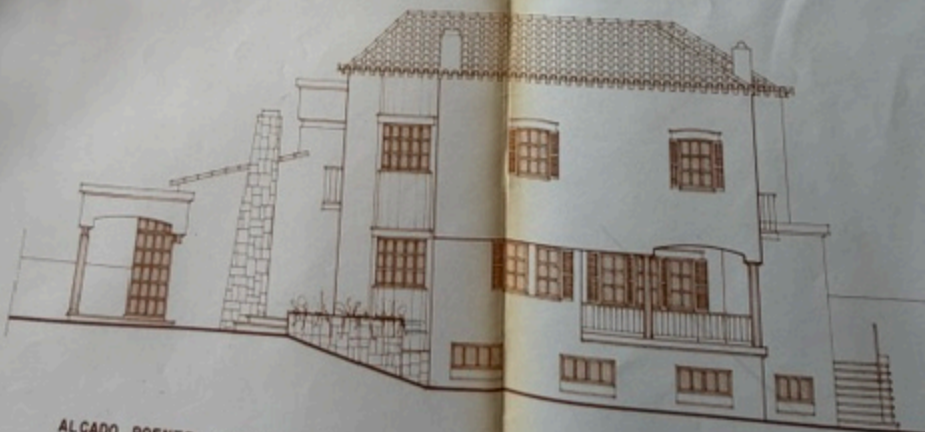
ALÇADO POENTE (PLANIFICADO)
