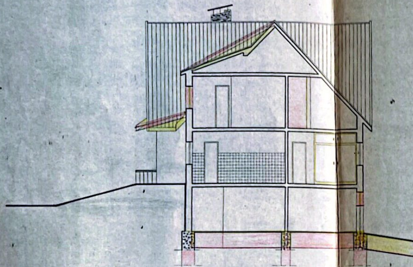
Corte A-B
