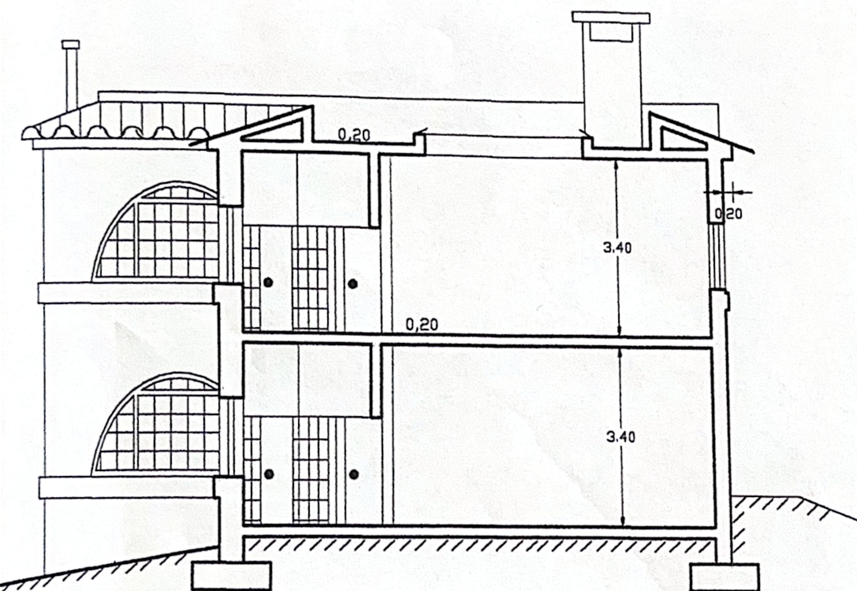
CORTE AB
