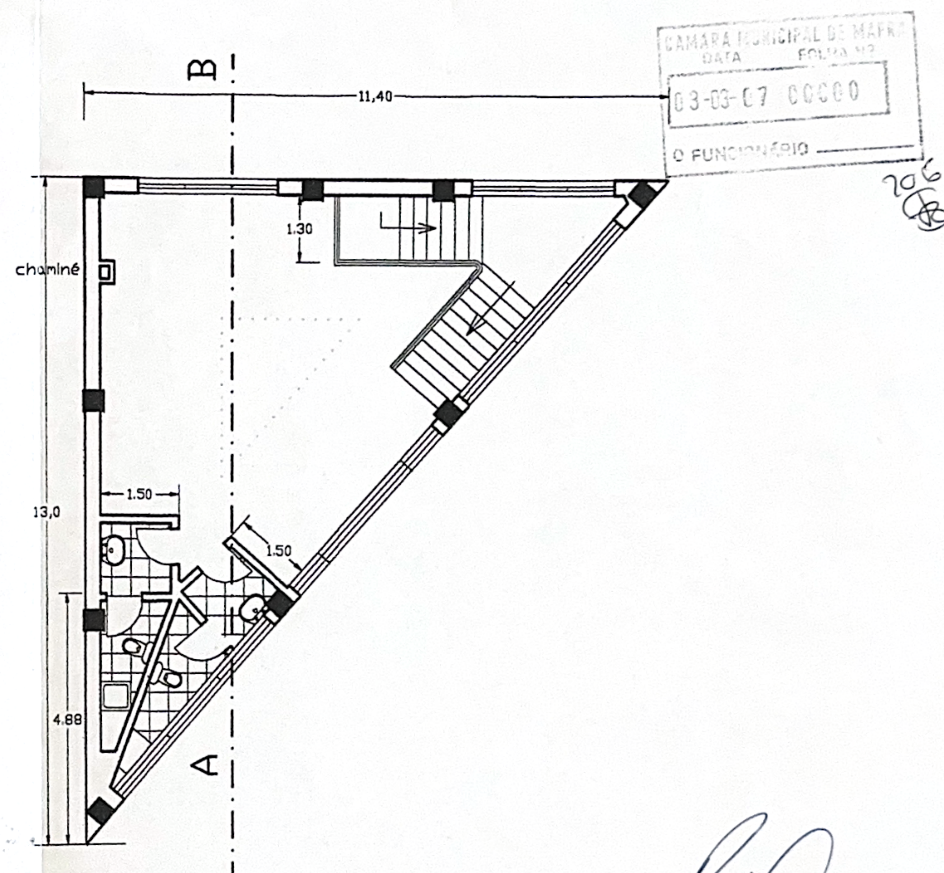
PLANTA DO 2º PISO
