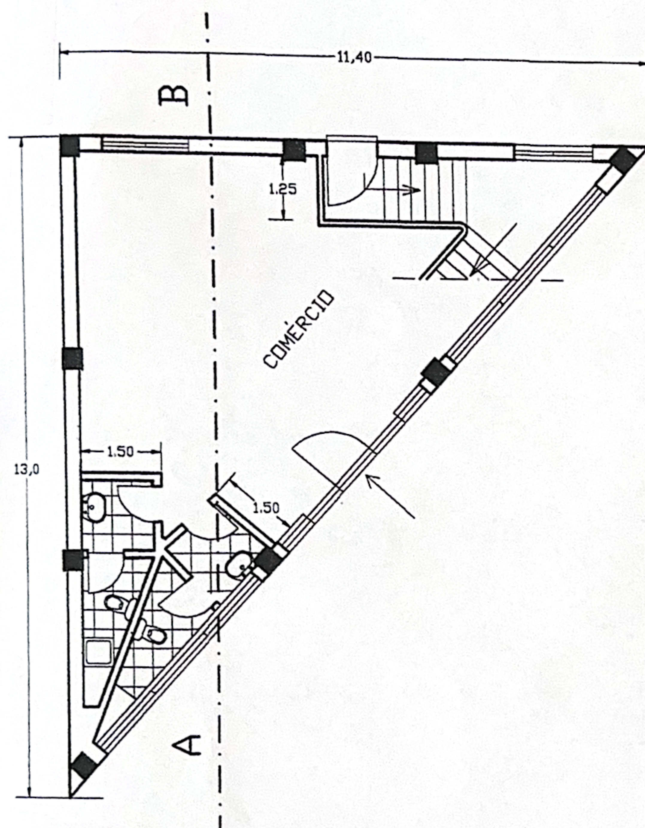
PLANTA DO 1º PISO
