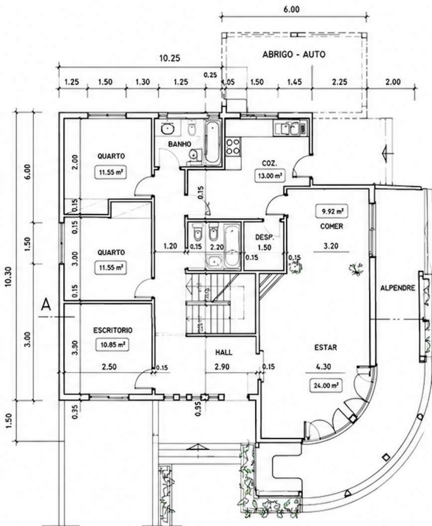
PLANTA R/C
