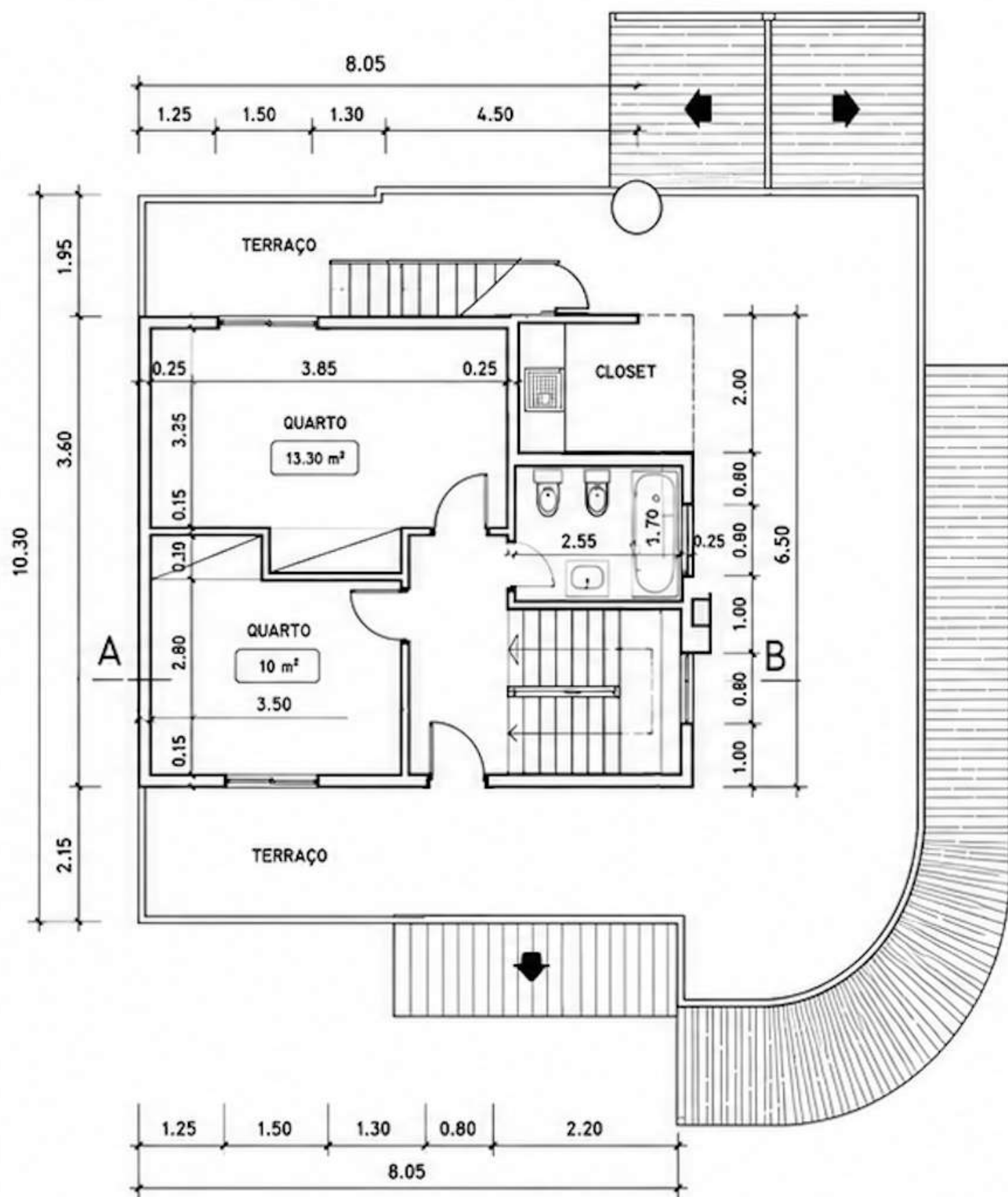
1º ANDAR
