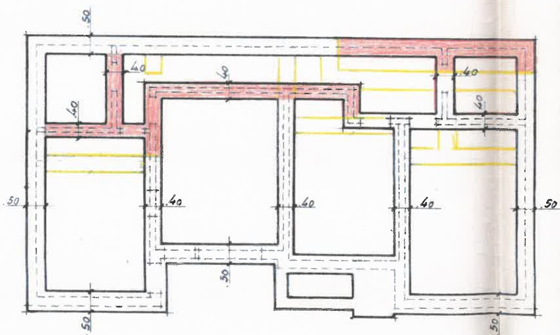
FUNDAÇÕES
