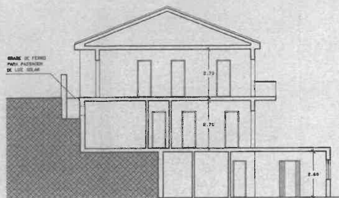
CORTE B-B
