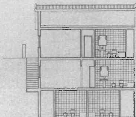
CORTE A-A
