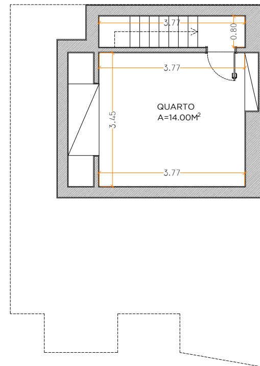
Planta Piso 01
