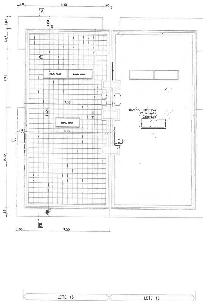
PLANTA DA COBERTURA
