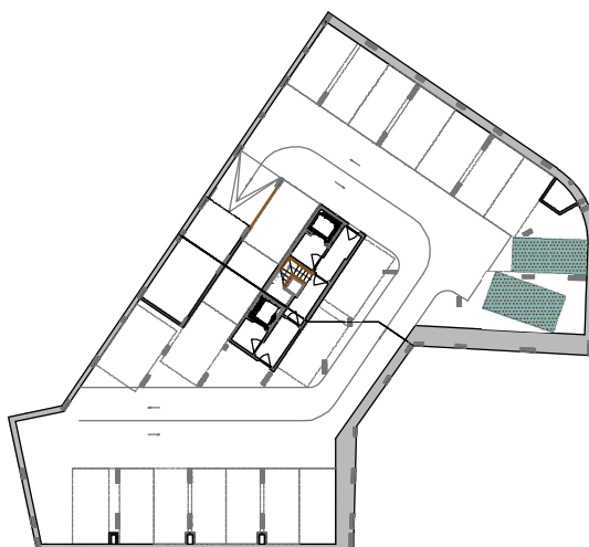
PLANTA DO PISO -1 - ESTACIONAMENTO T3 FRAÇÃO H
