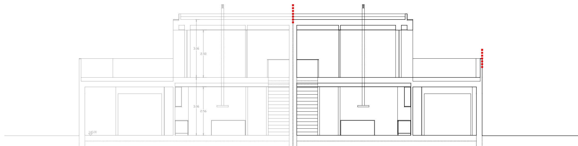
corte c3, escala 1/100
