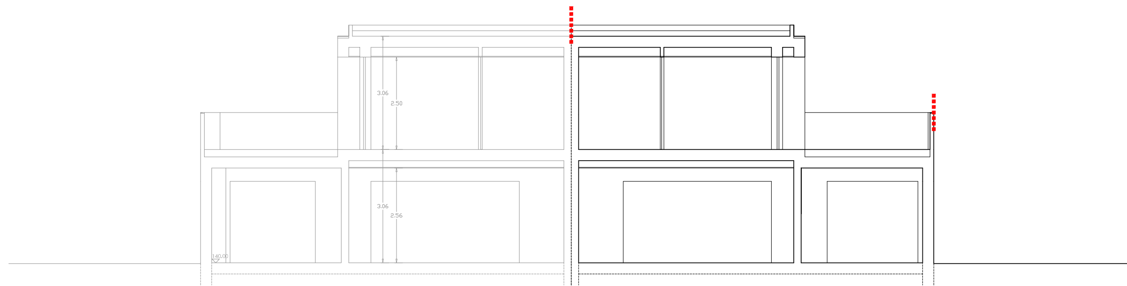
corte c4, escala 1/100
