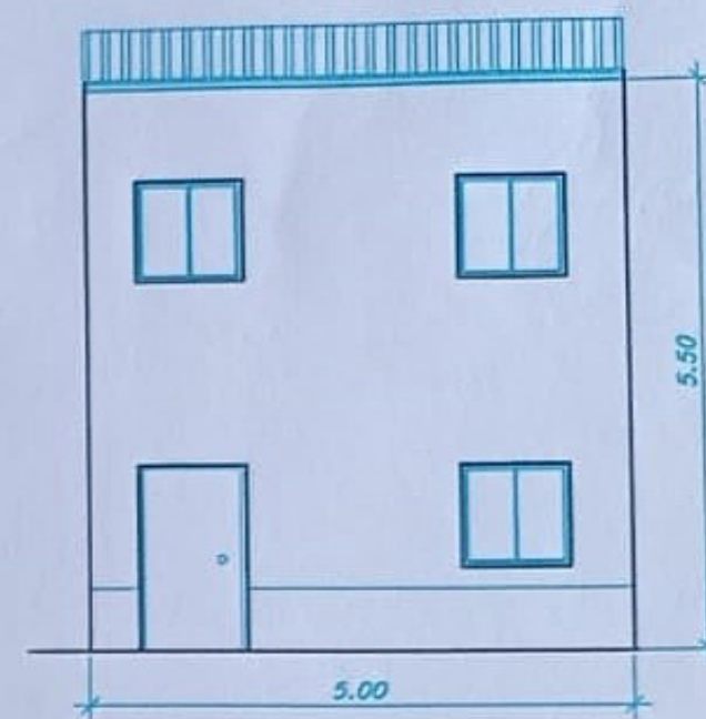
ALÇADO PRINCIPAL
