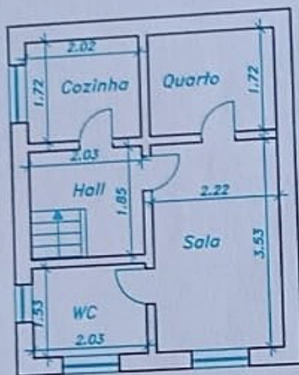
PLANTA DO 1º ANDAR
