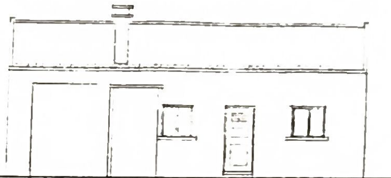
ALCADO POSTERIOR
