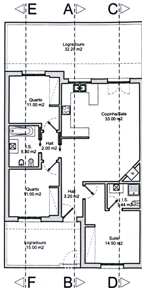
PLANTA DE PISO (apresentação)
