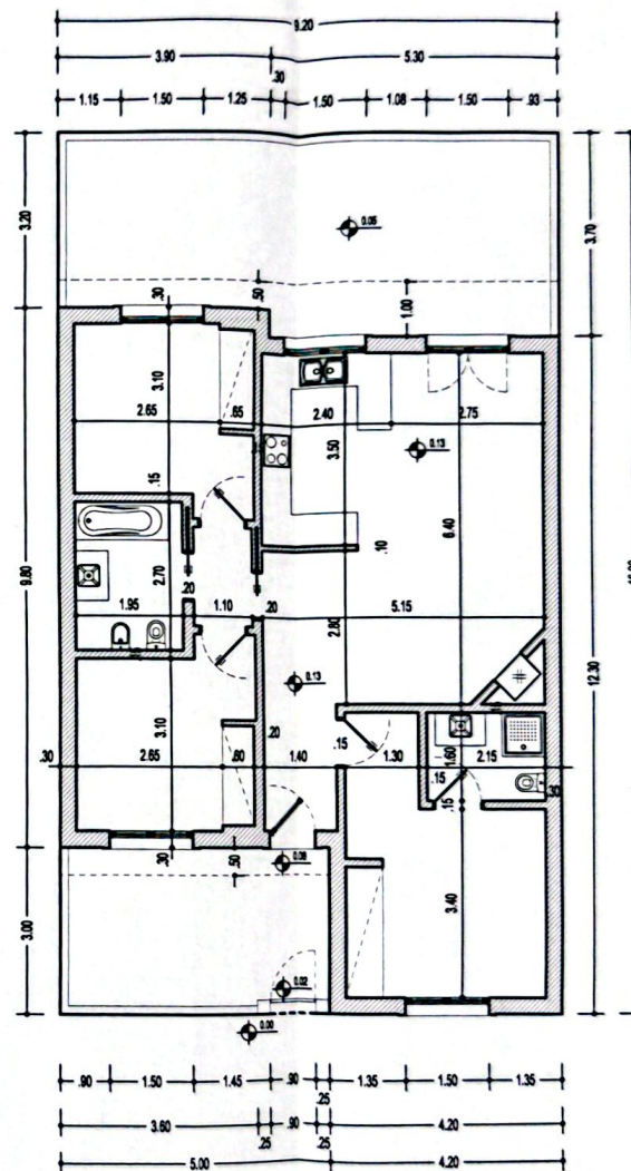
PLANTA DE PISO (cotada)
