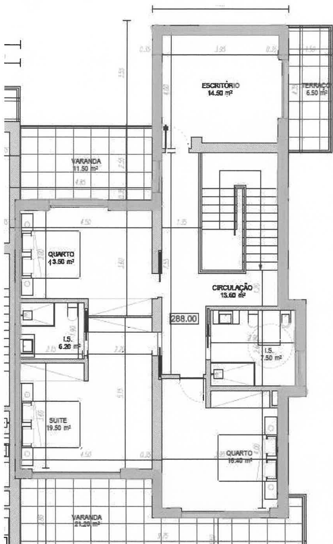
FTH/Anexo n.º 5 – Planta Simplificada da Habitação
