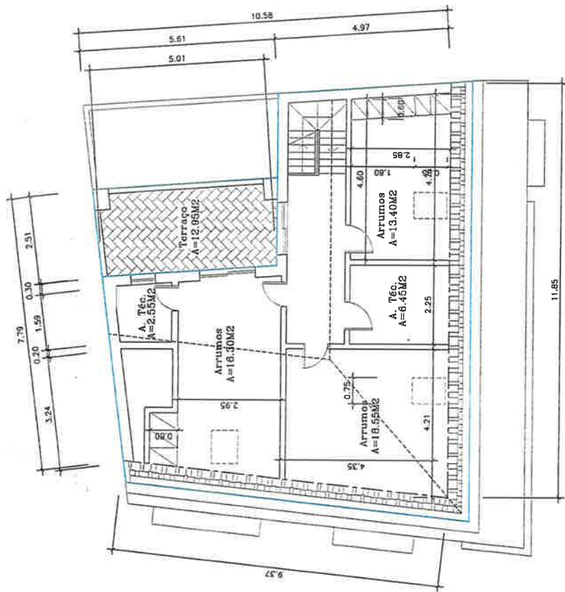
PLANTA - ESTEIRA (Habitação)
