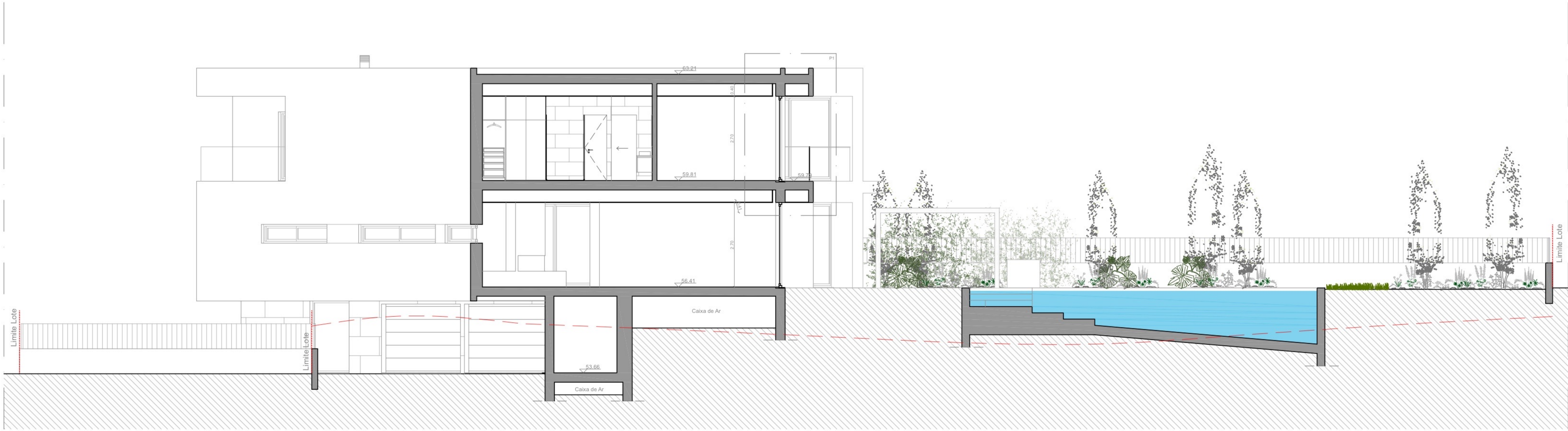
CORTE EF
