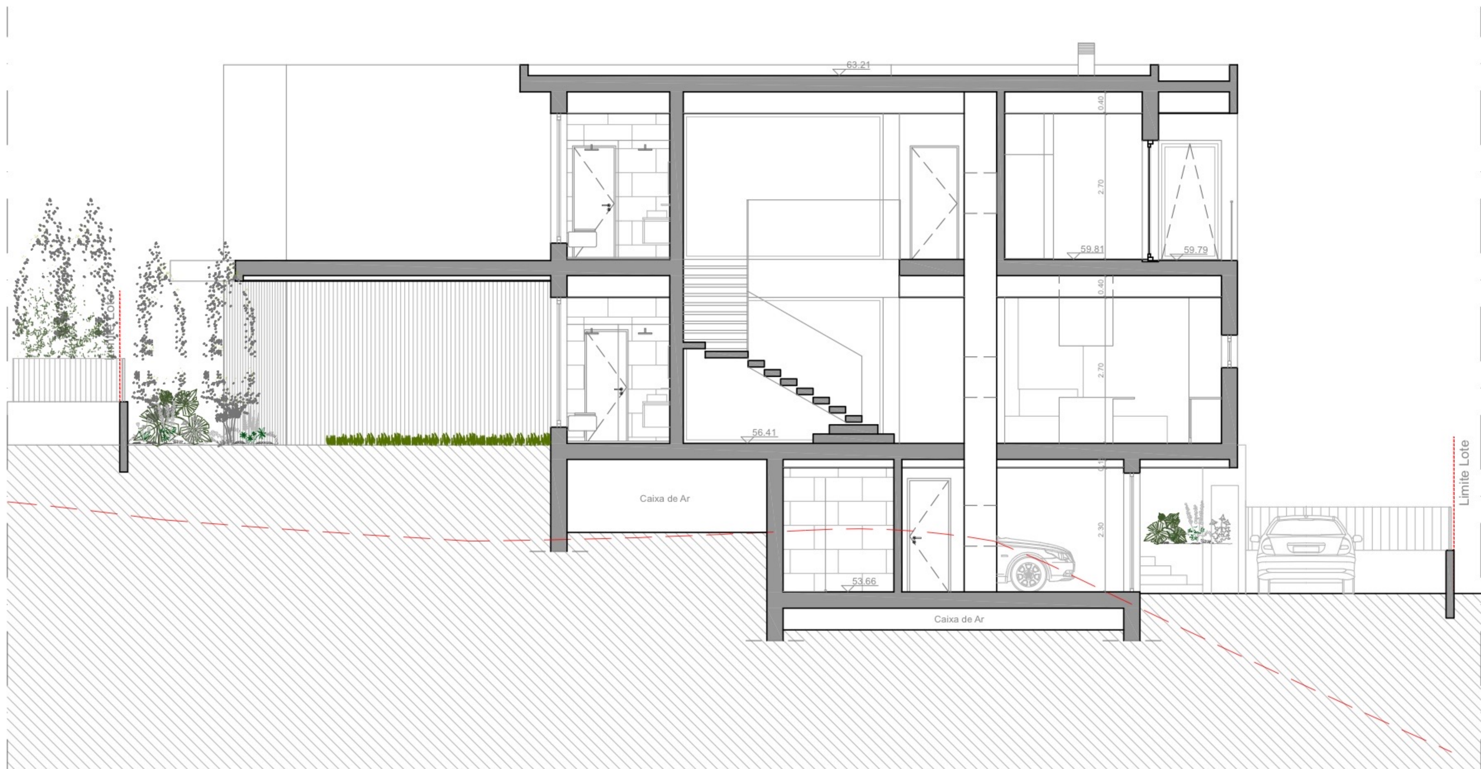
Corte CD
