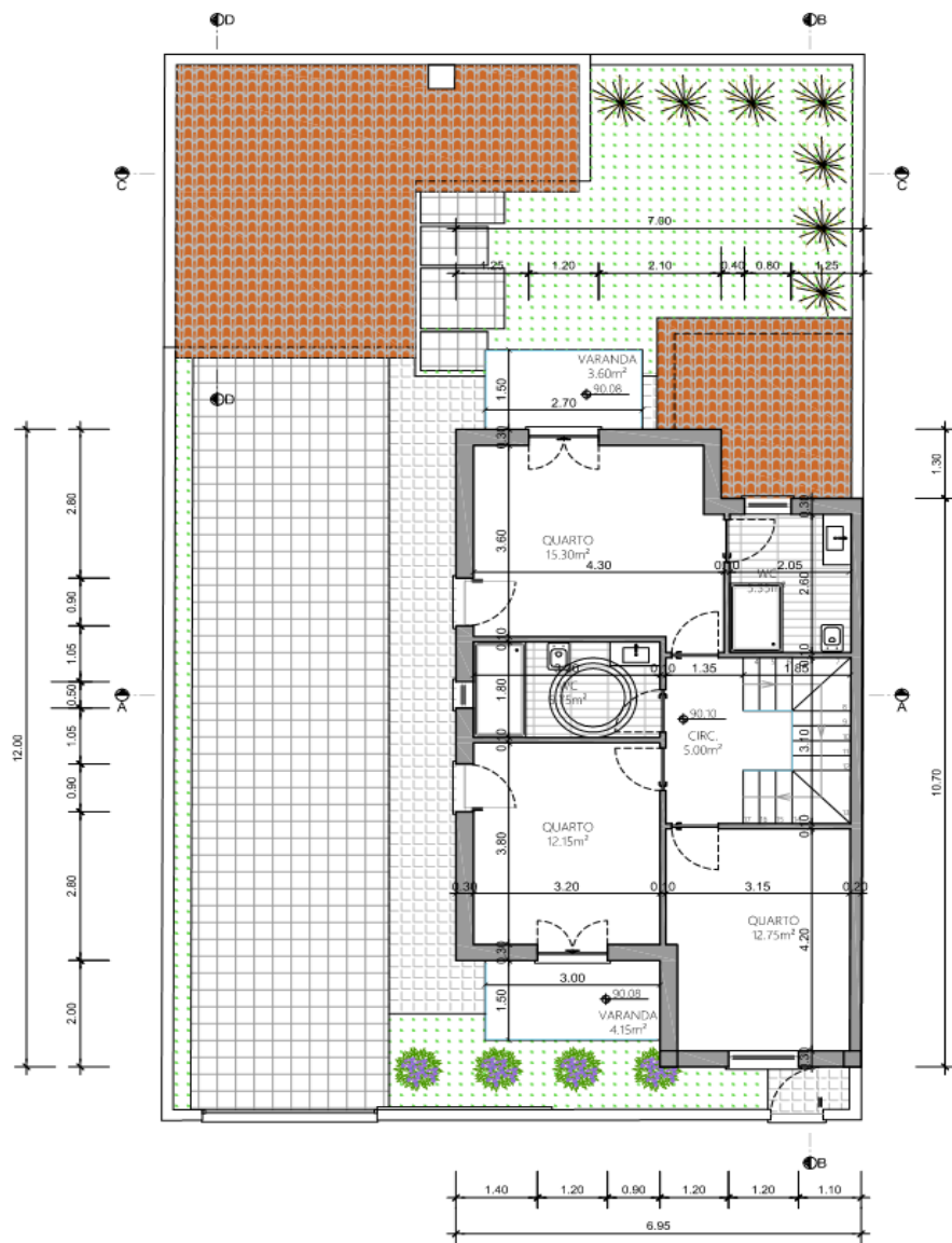
PLANTA DO PISO 1
