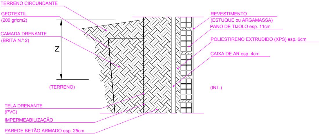
"LIGAÇÃO DA FACHADA COM PAVIMENTOS TÉRREOS e PAREDES ENTERRADAS"
