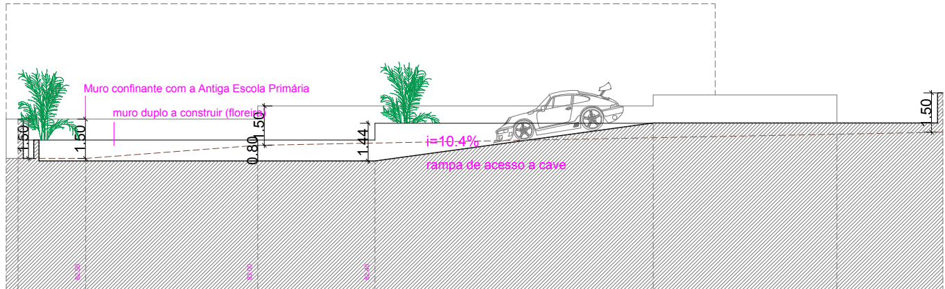
Perfil do muro confinante com a Antiga Escola Primária
