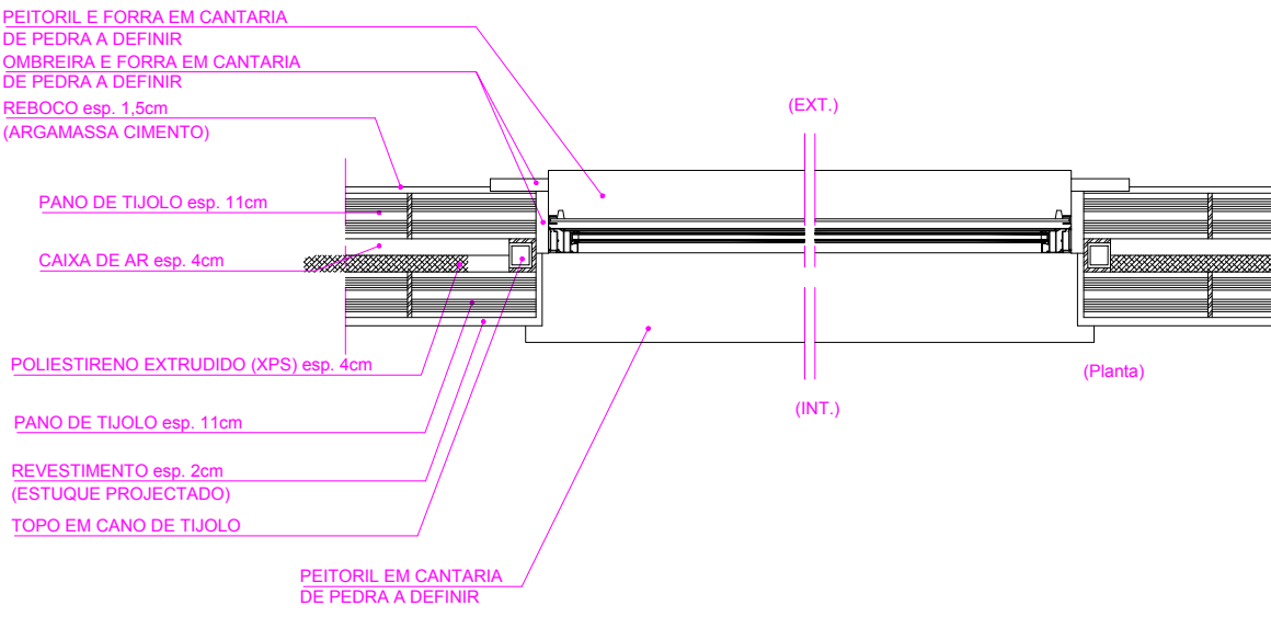
"LIGAÇÃO ENTRE DUAS PAREDES VERTICAIS"
