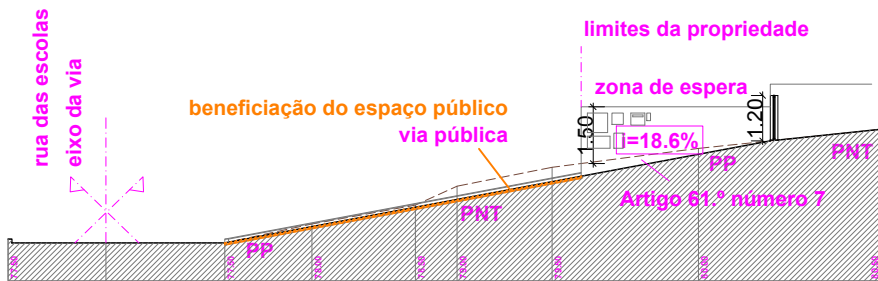
Perfil do muro alçado lateral esquerdo
