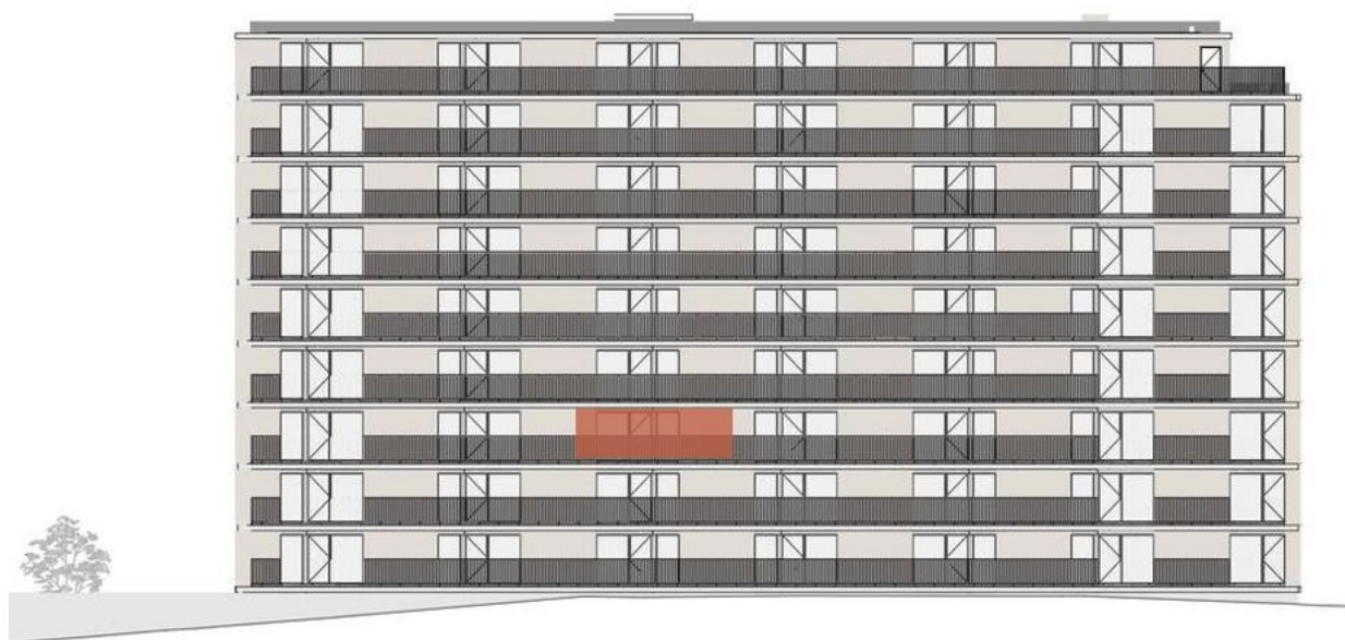
ALÇADO PRINCIPAL
