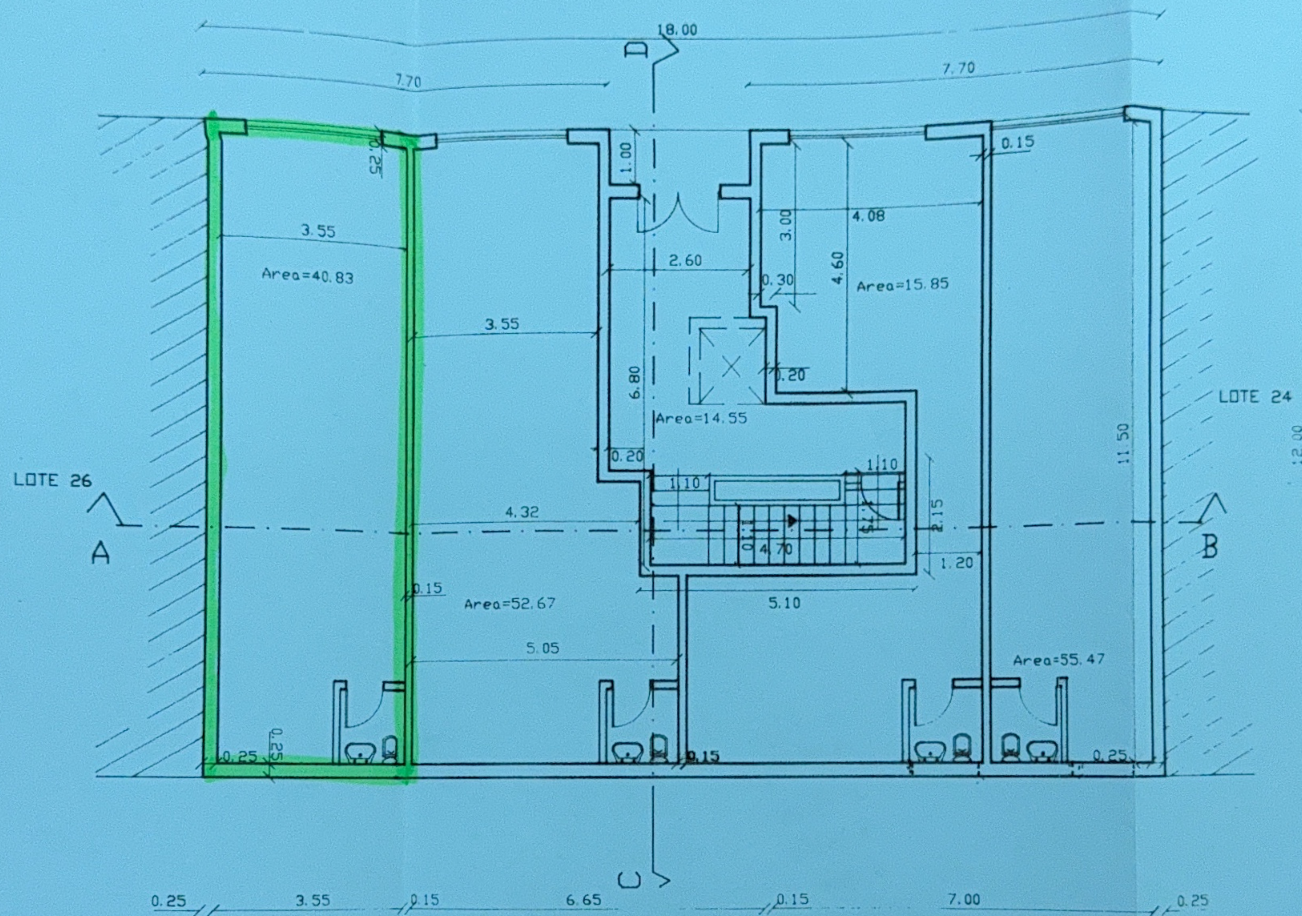
PLANTA DA CAVE
