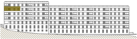
ALÇADO NOROESTE
