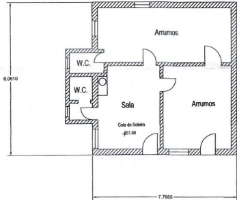
Planta do 1º Piso
