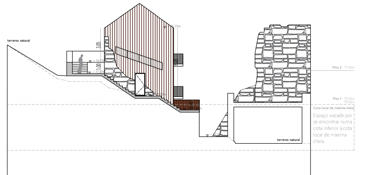
CORTE 12 - Transversal 5
