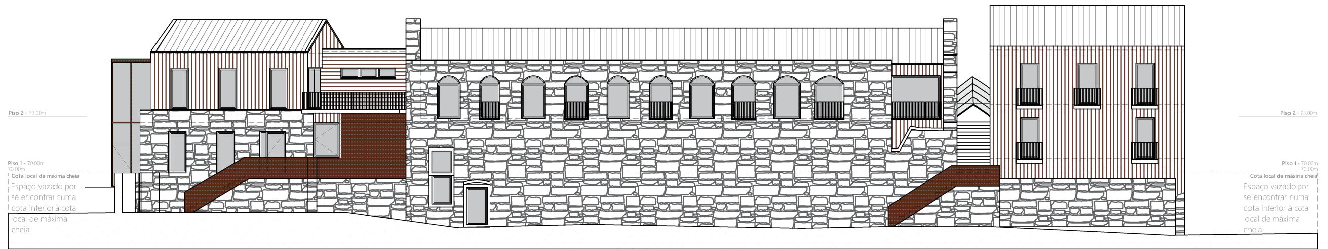
ALÇADO PRINCIPAL
