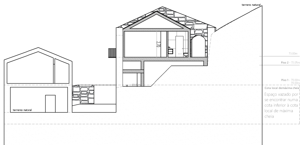
CORTE 10 - Transversal 3
