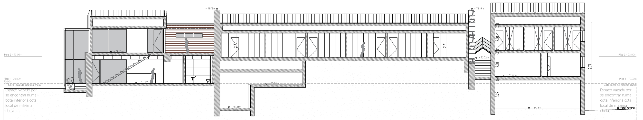
CORTE 06 - Longitudinal 2
