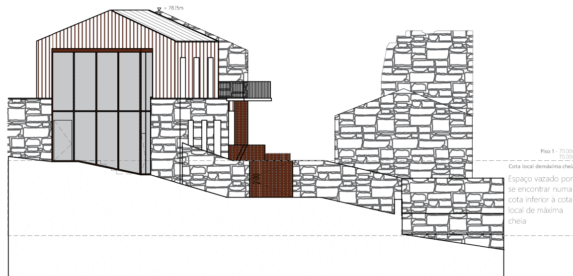
ALÇADO LATERAL ESQUERDO
