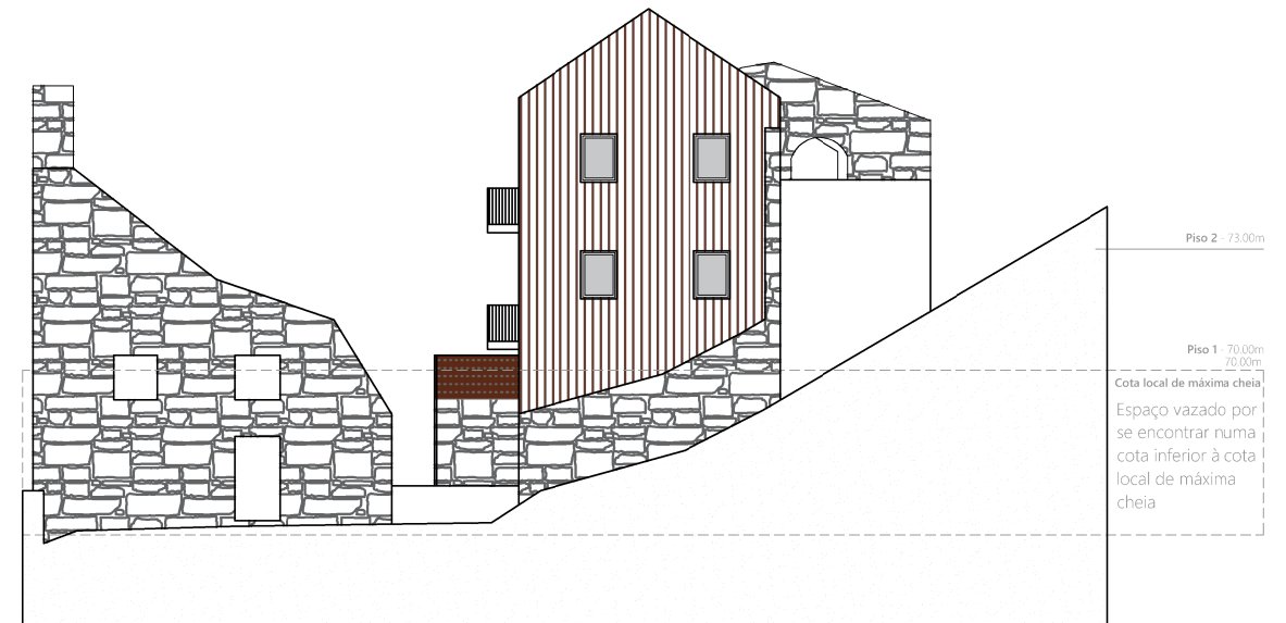
ALÇADO LATERAL DIREITO
