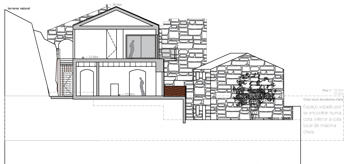
CORTE 08 - Transversal 1
