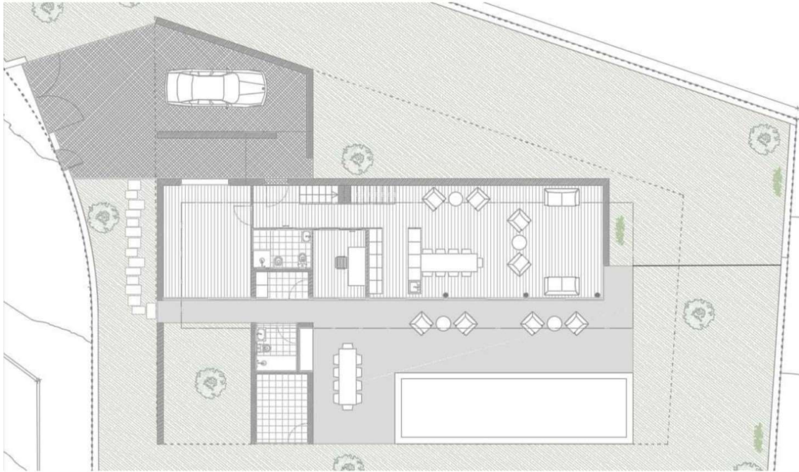
Planta de piso 1
