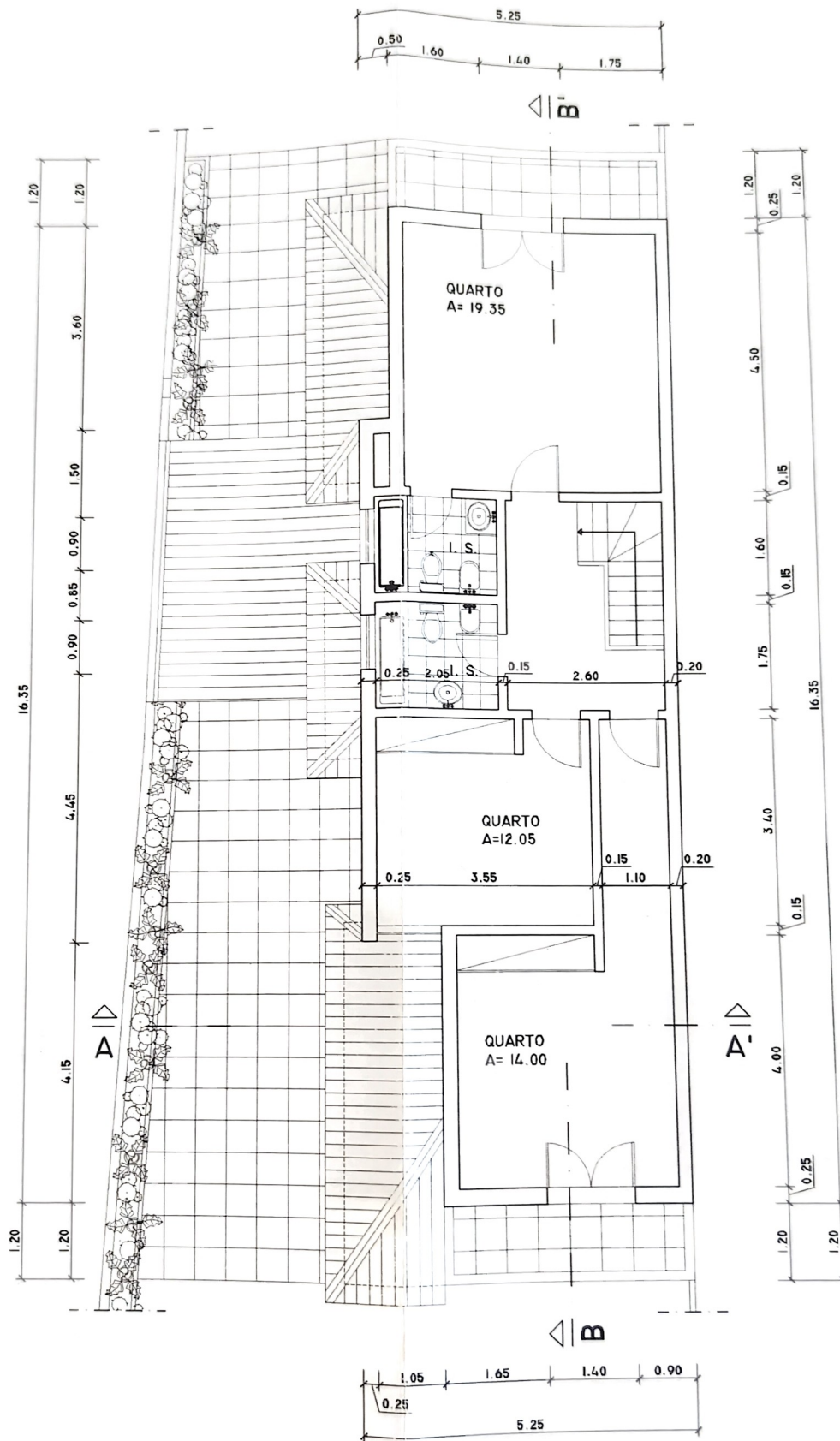
PLANTA PISO I
