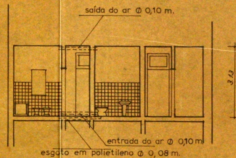
CORTE POR A-B
