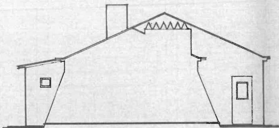
ALÇADO SUL
