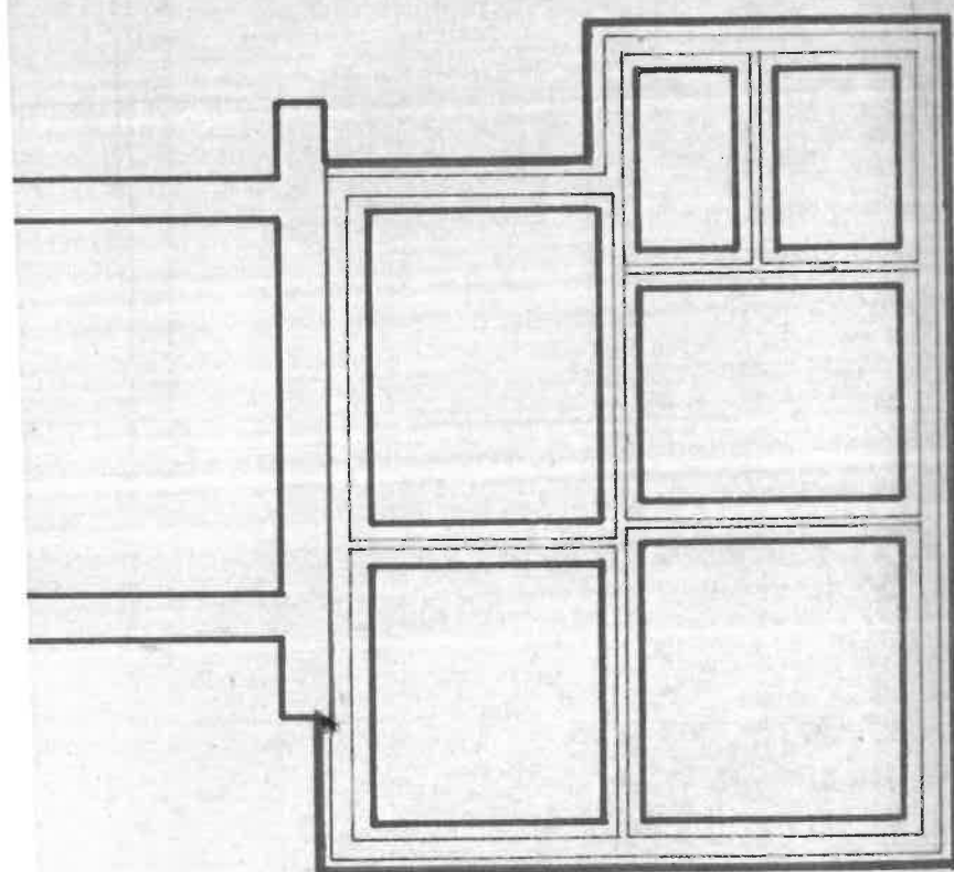
FUNDAÇÕES
