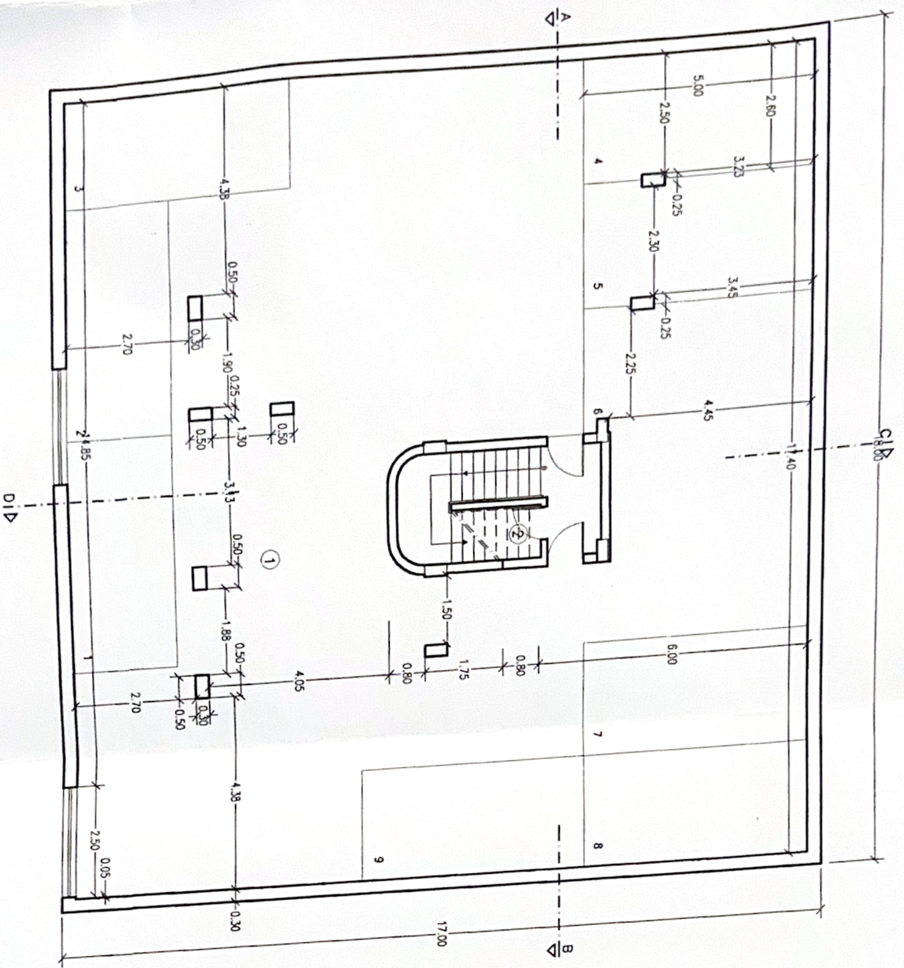
PLANTA DA CAVE
