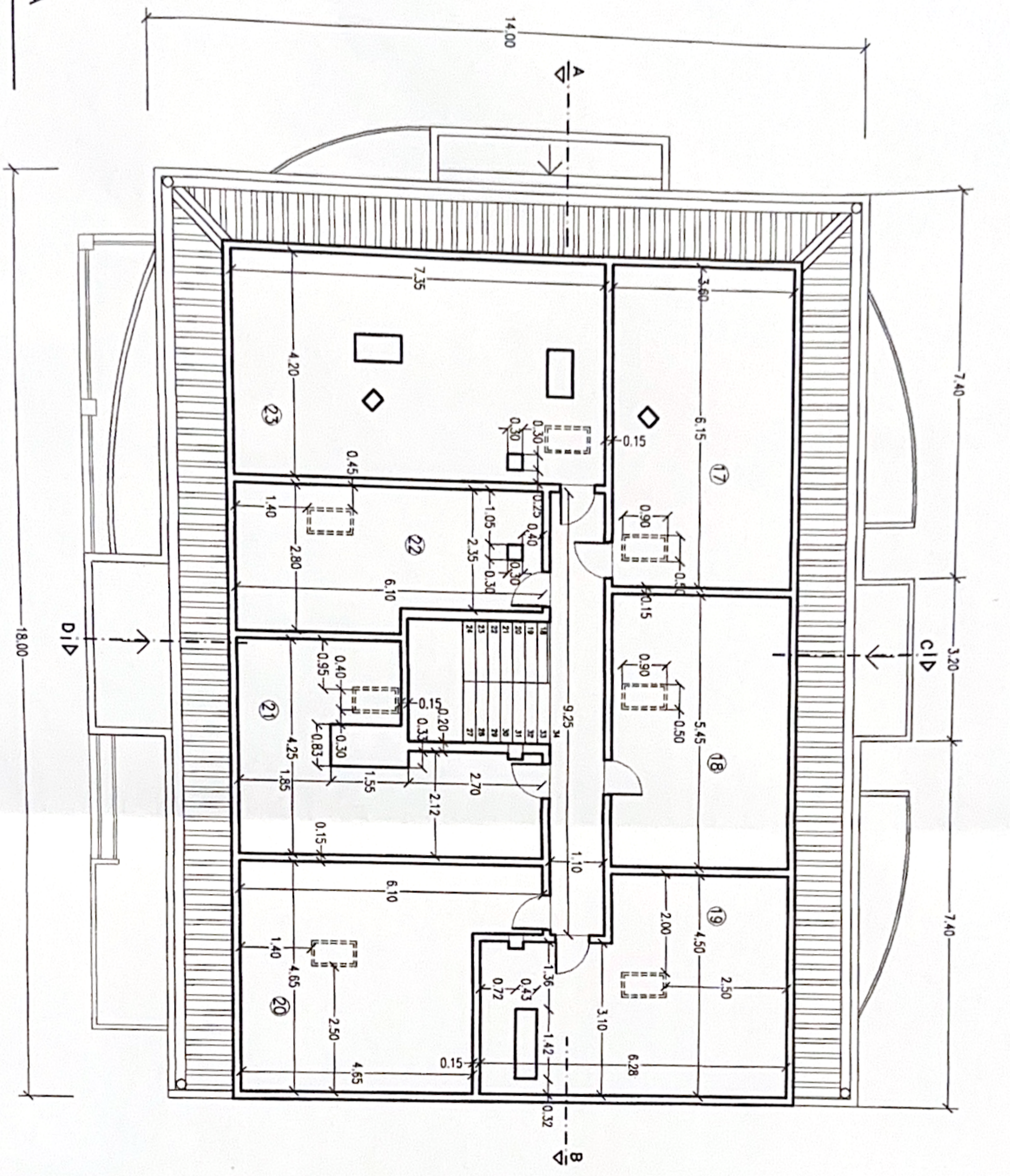
PLANTA DO SOTÃO
