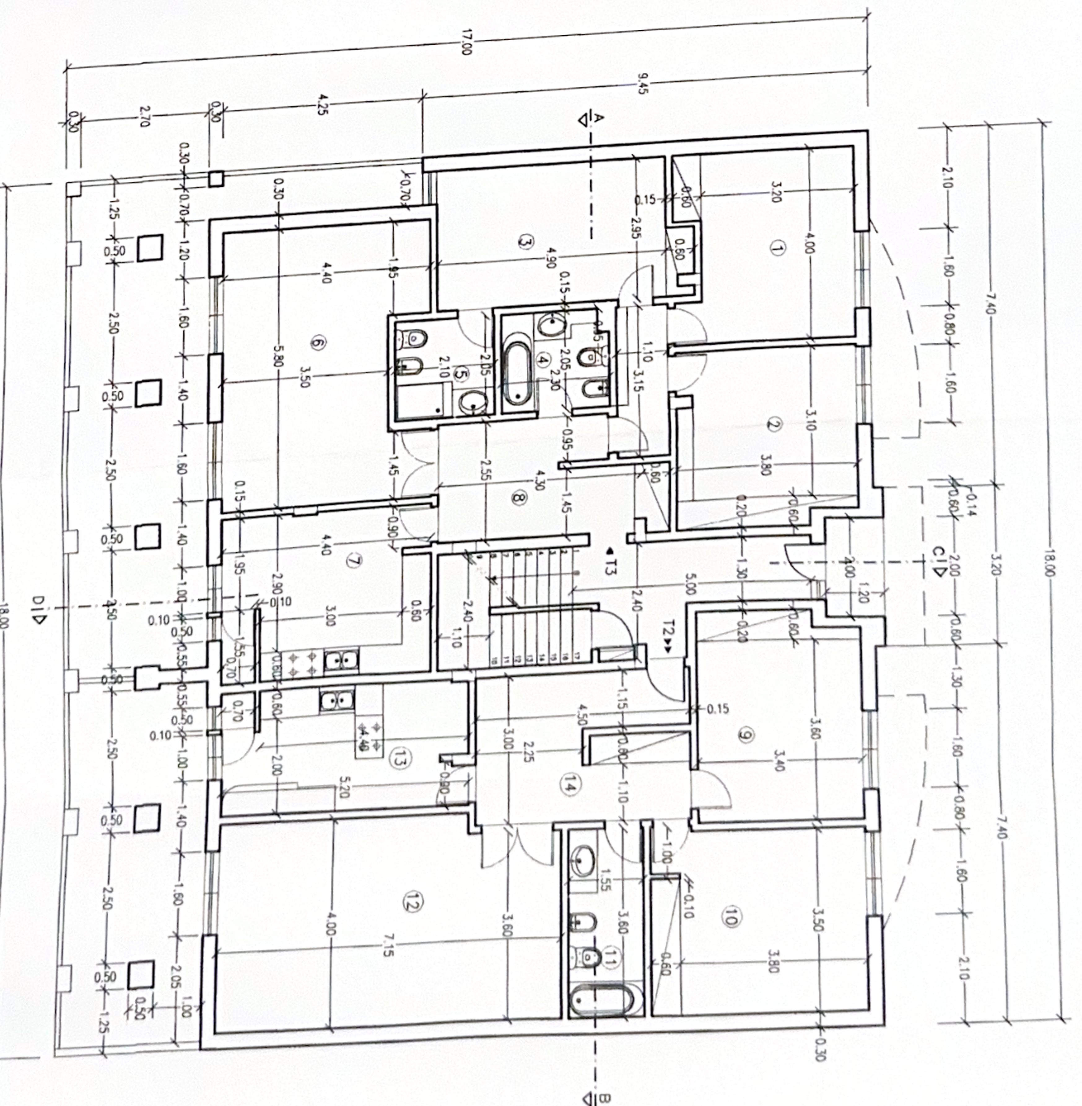
PLANTA DO PISO 1
