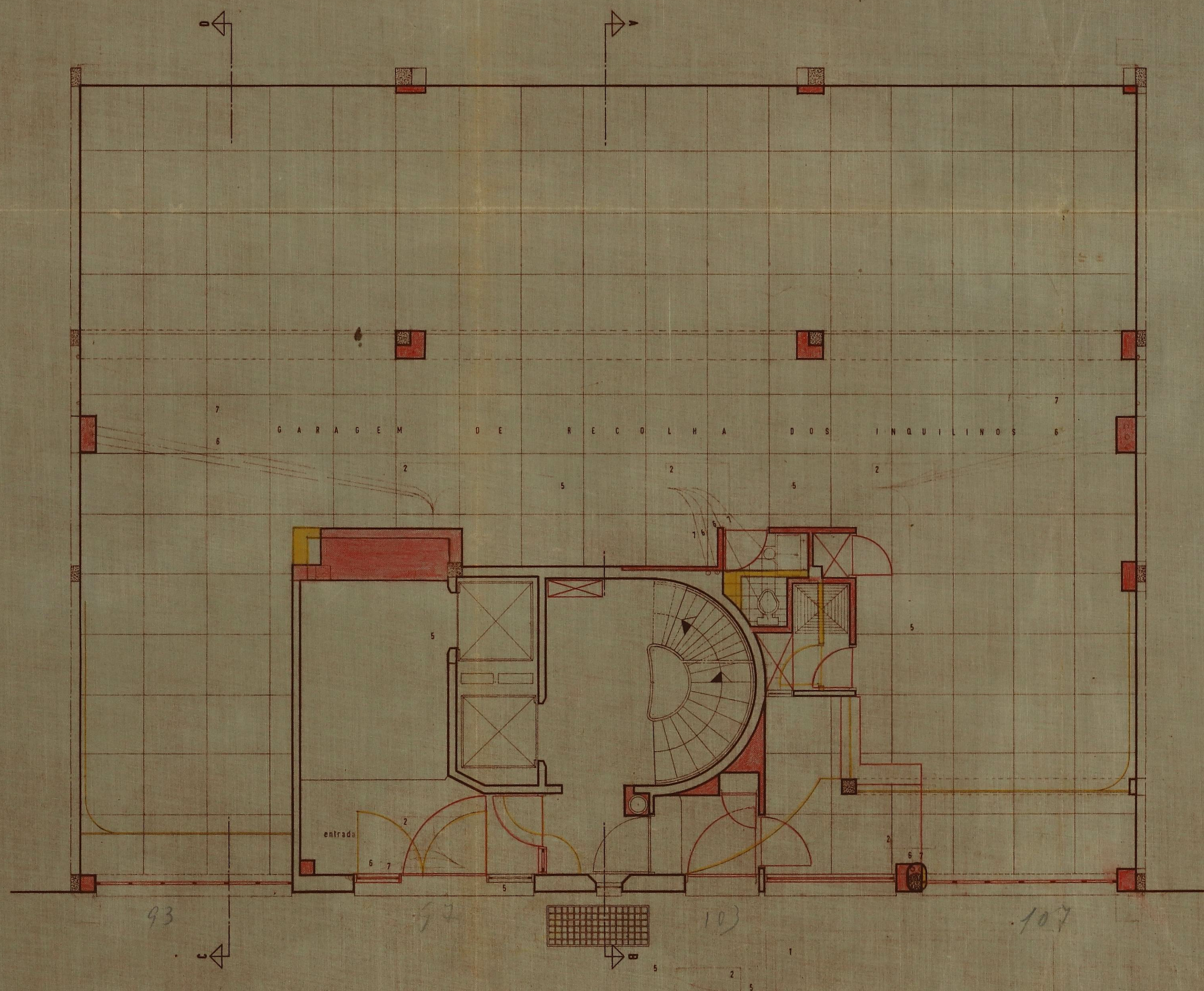
PLANTA DO RÉS-DO-CHÃO
