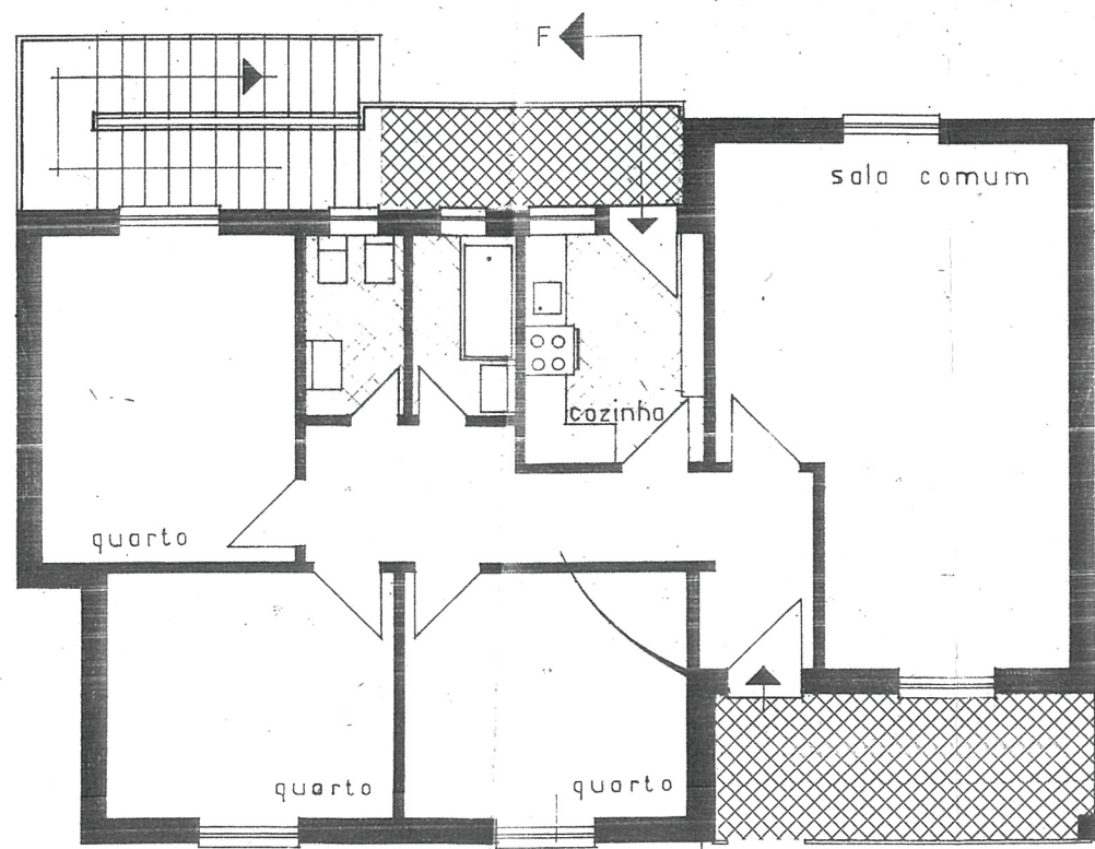
RÉS-DO-CHÃO
