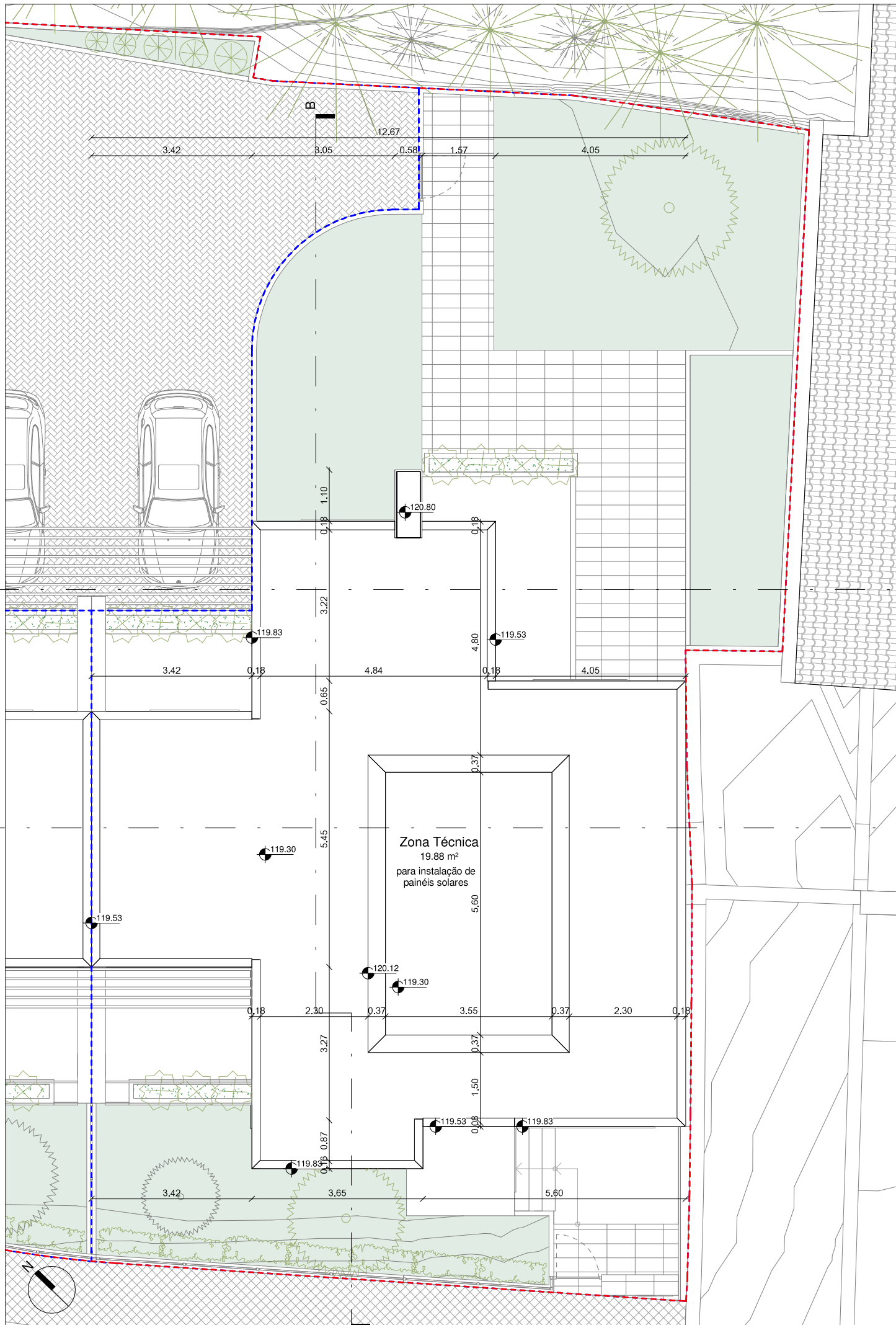
Planta de Coberturas - Moradia 2 (Fração B)
