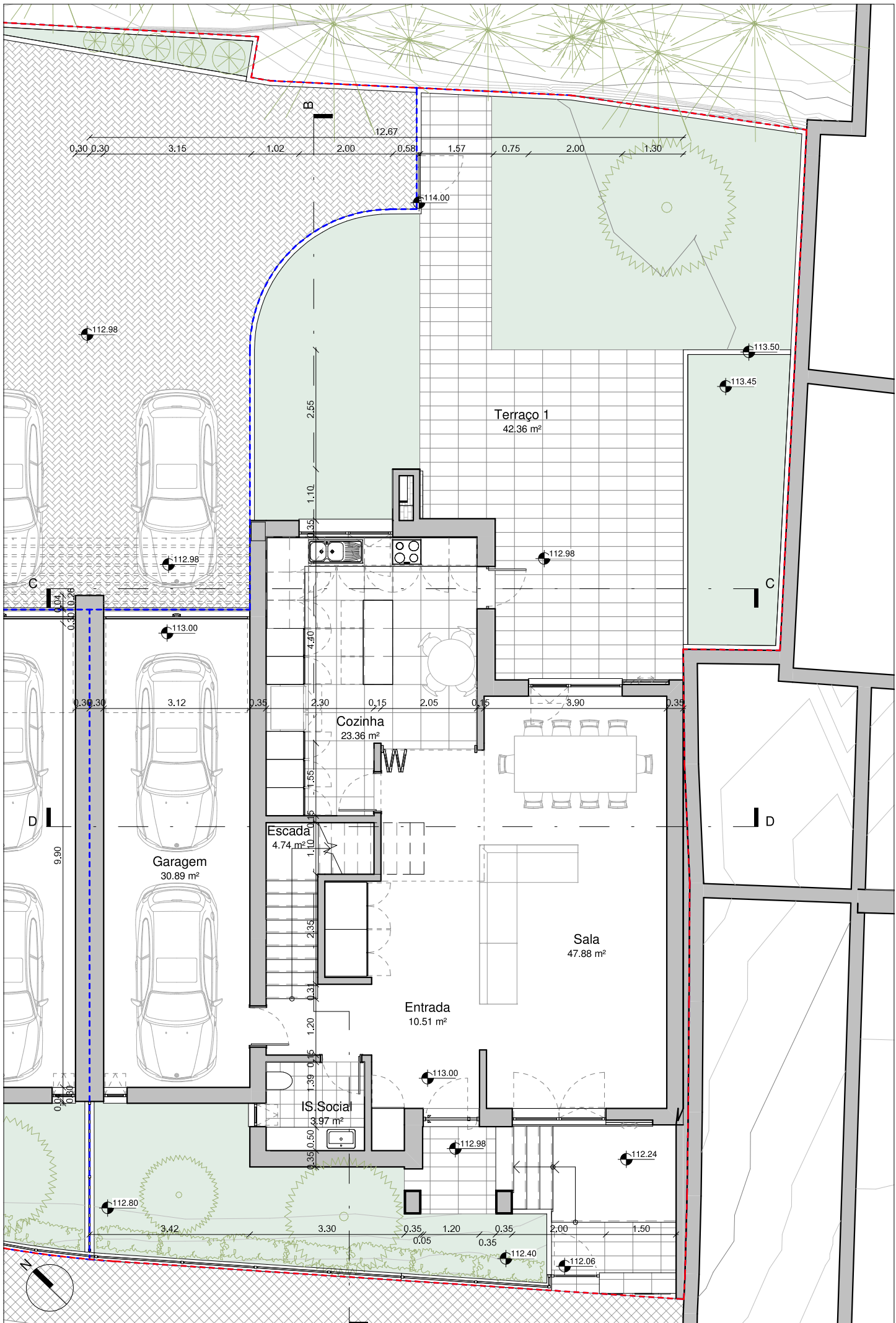
Planta do Piso Térreo - Moradia 2 (Fração B)
