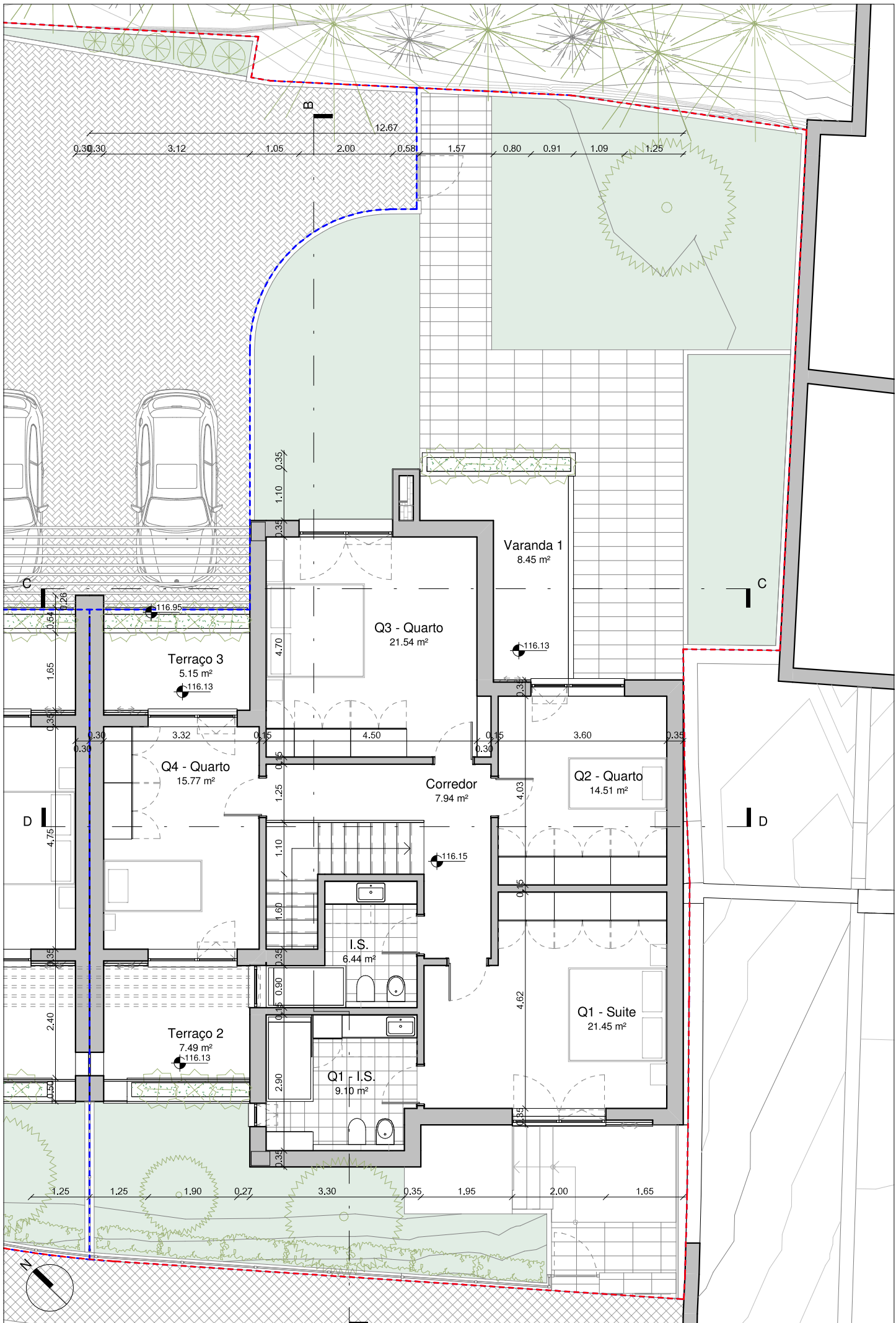
Planta do 1º Andar - Moradia 2 (Fração B)
