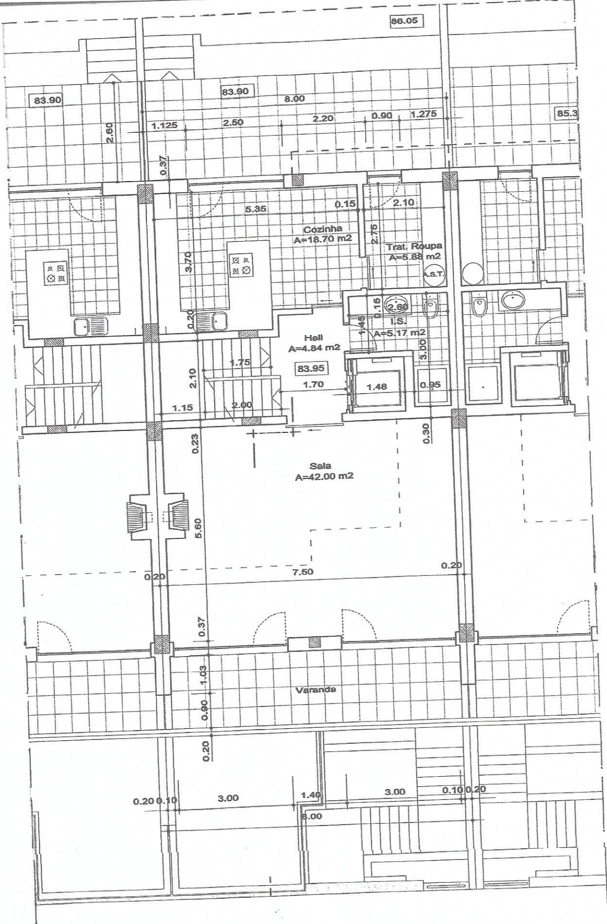
PLANTA DO PISO 1
