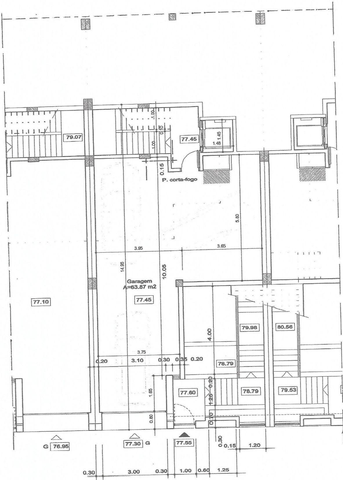
PLANTA DO PISO - 2
