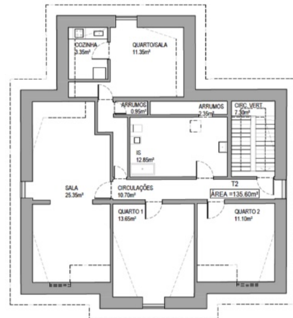
PLANTA PISO 2
