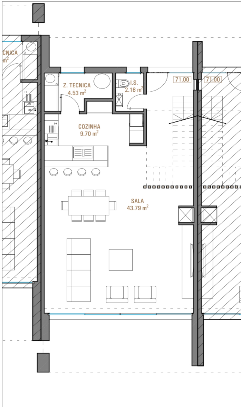
PLANTA DO PISO TERREO
