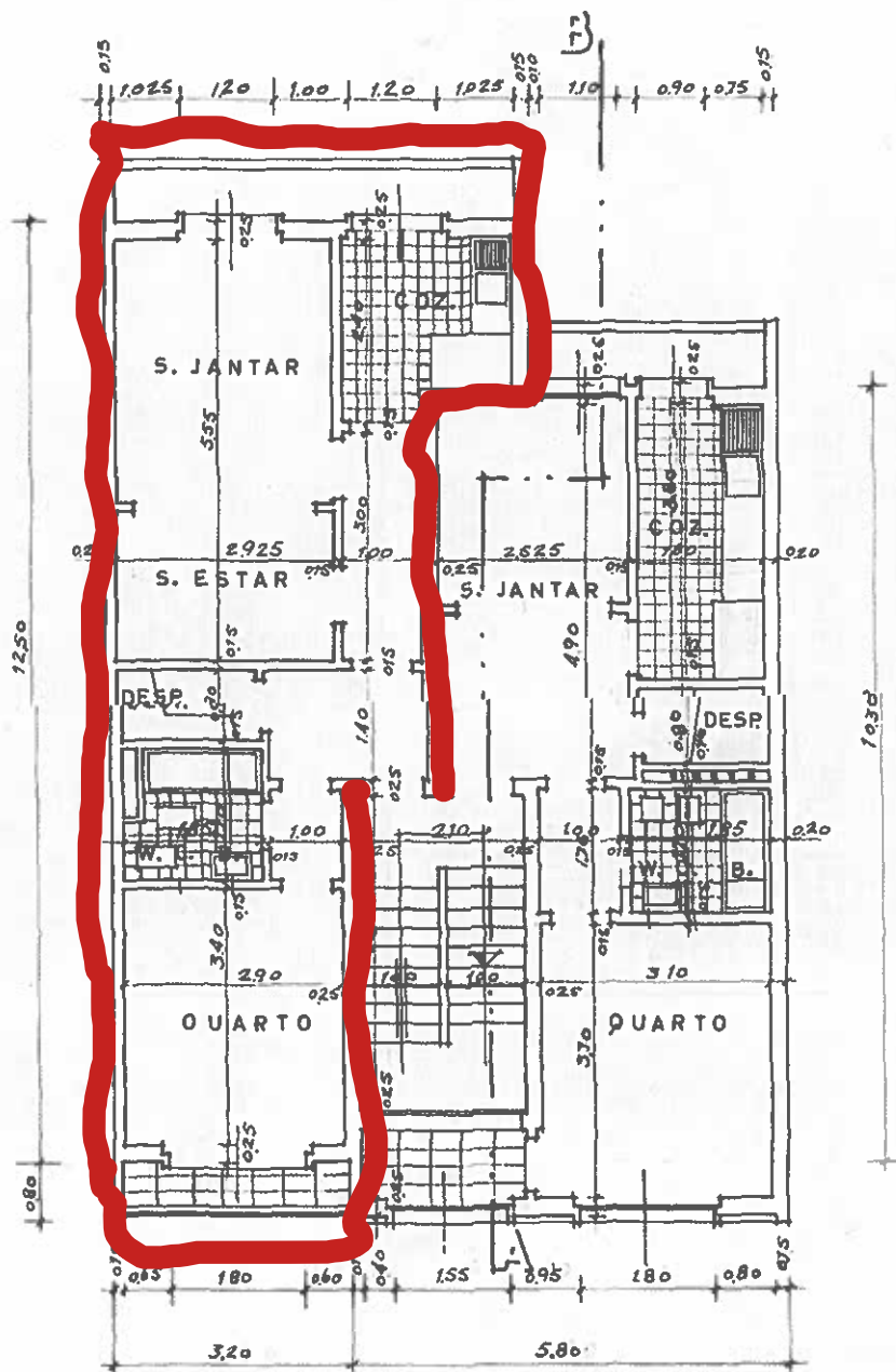
PLANTA DOS ANDARES
